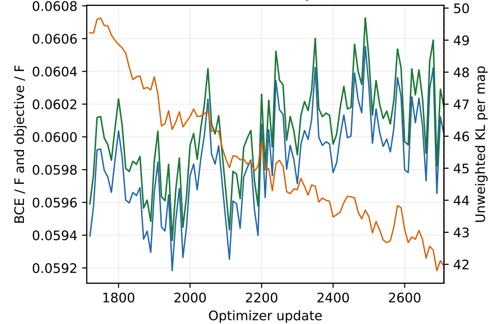
Posterior-mean validation · updates 1711-2710
