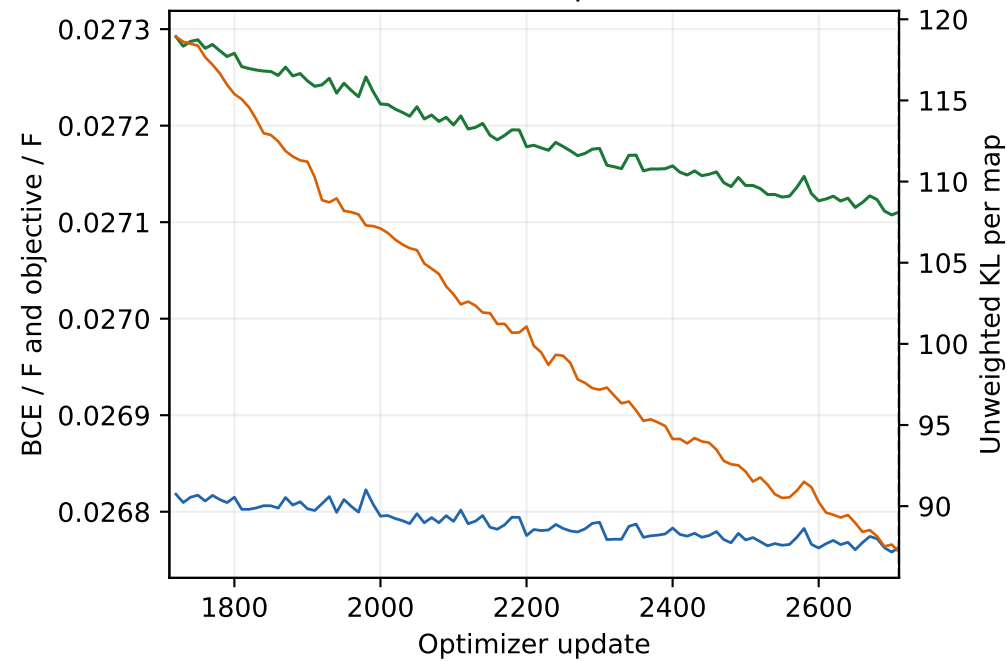
Posterior-mean train · updates 1711-2710
