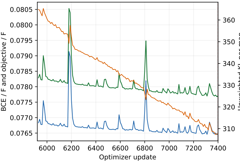
Posterior-mean train · updates 5921-7400
