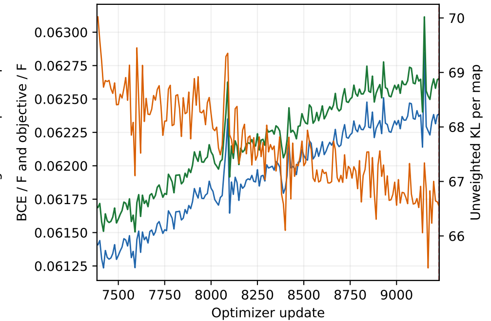
Posterior-mean validation · updates 7385-9230
