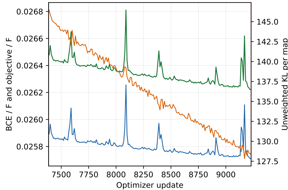
Posterior-mean train · updates 7385-9230
