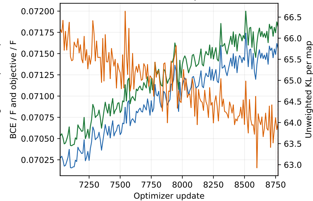
Posterior-mean validation · updates 7017-8770
