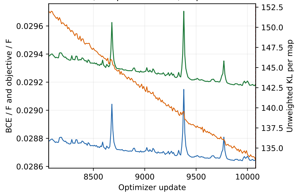
Stochastic train (10-update means) · updates 8065-10080
