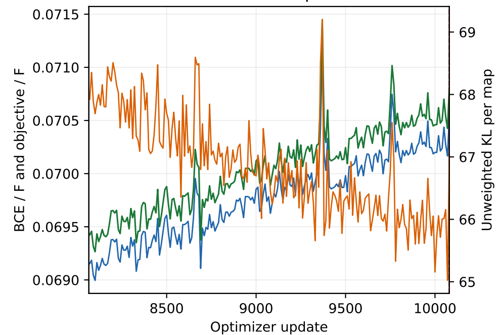
Posterior-mean validation · updates 8065-10080
