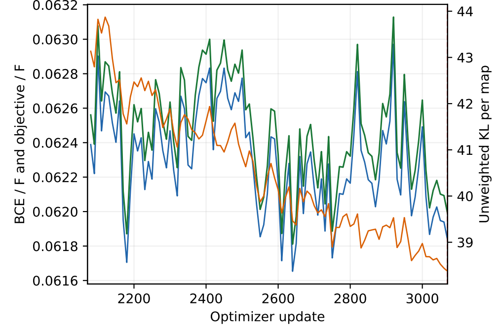
Posterior-mean validation · updates 2071-3070
