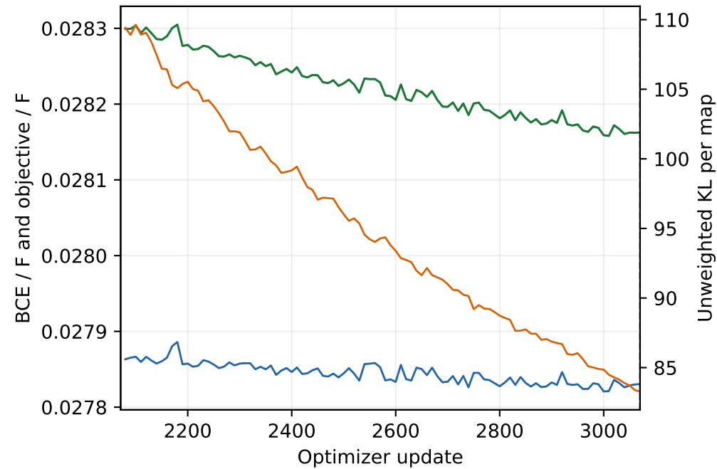
Posterior-mean train · updates 2071-3070
