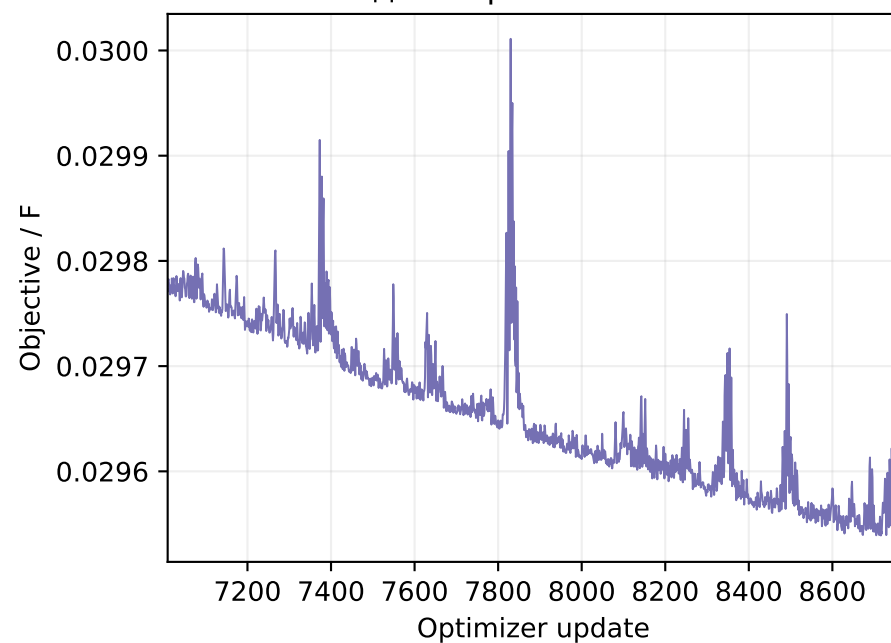
Последние updates: 7009-8760
