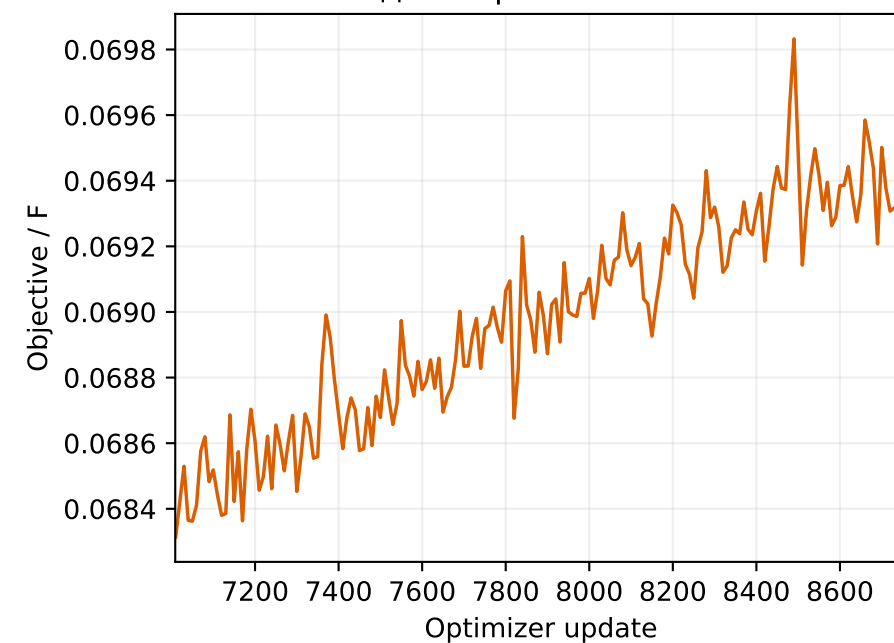
Последние updates: 7009-8760
