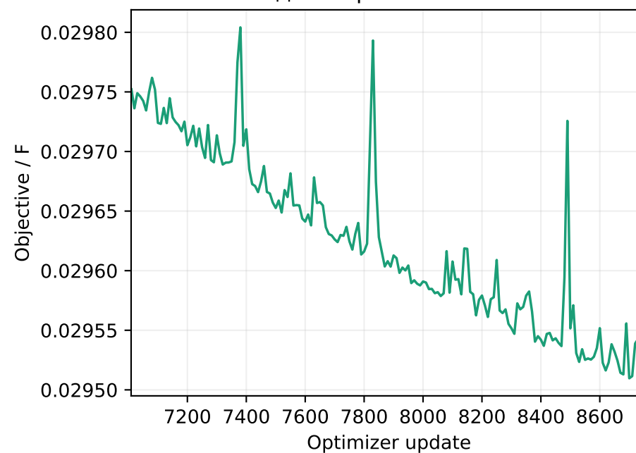
Последние updates: 7009-8760
