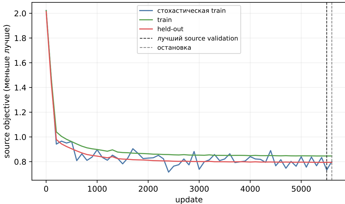
gnn_flow, seed 4100: source-only обучение
