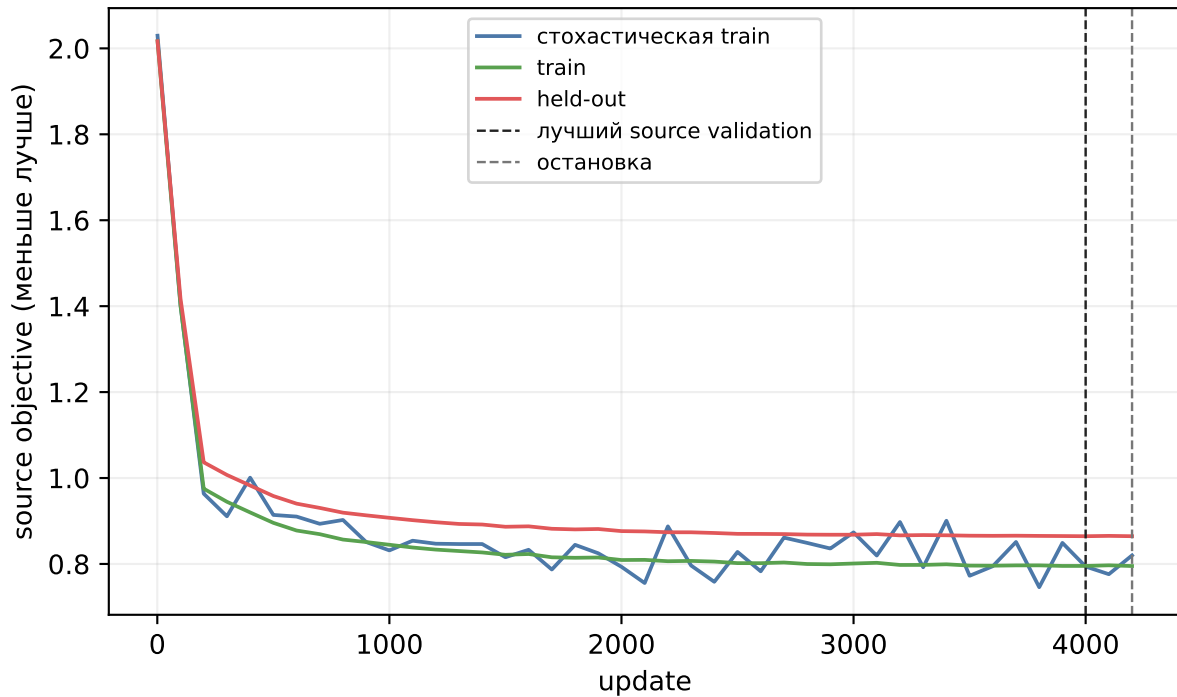
gnn_flow, seed 4103: source-only обучение
