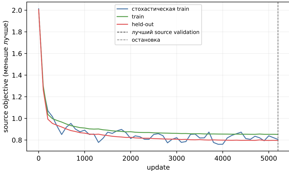
gnn_flow, seed 4104: source-only обучение
