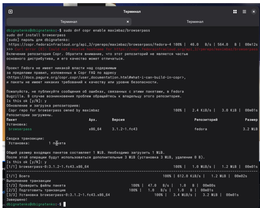
Рис. 4.9: Установка browserpass
