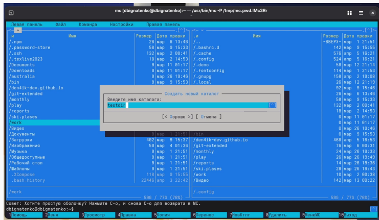
Рис. 6: Создание каталога
