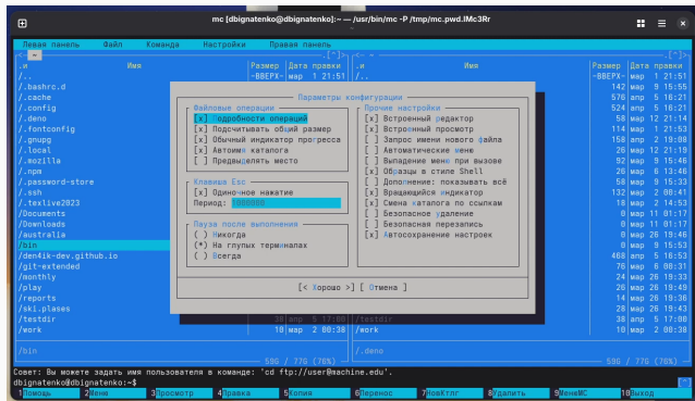
Рис. 9: Диалог «Конфигурация»
