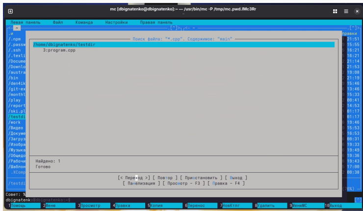
Рис. 8: Результат поиска
