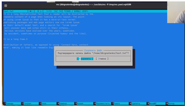
Рис. 12: Сохранение файла
