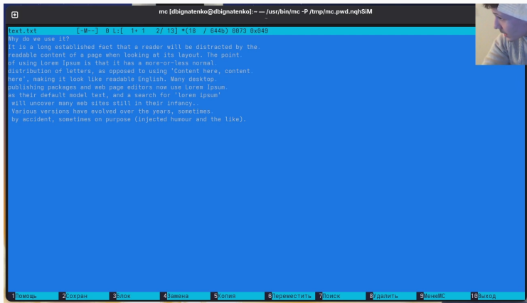
Рис. 10: Редактирование text.txt
