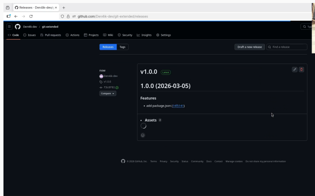
Рис. 11: Страница релизов
