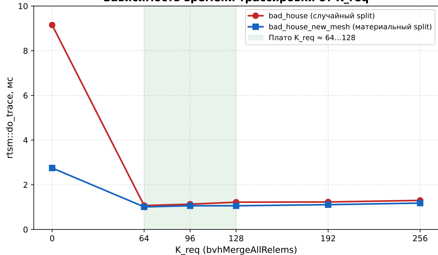
Зависимость времени трассировки от K_req
