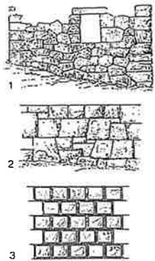
Mauerwerk der griechischen Antike 1 Polygonalmauerwerk 2 pseudoisodomes Quadermauerwerk 3 isodomes Quadermauerwerk
