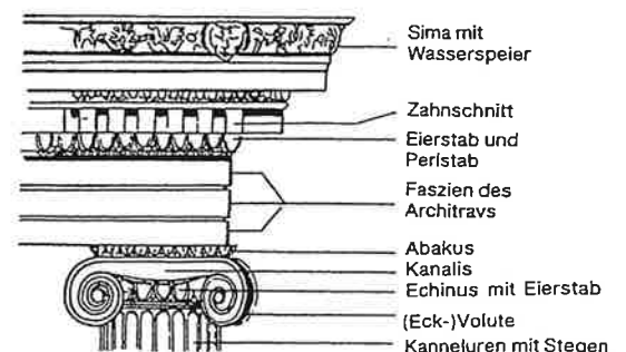
Die ionische Bauordnung
