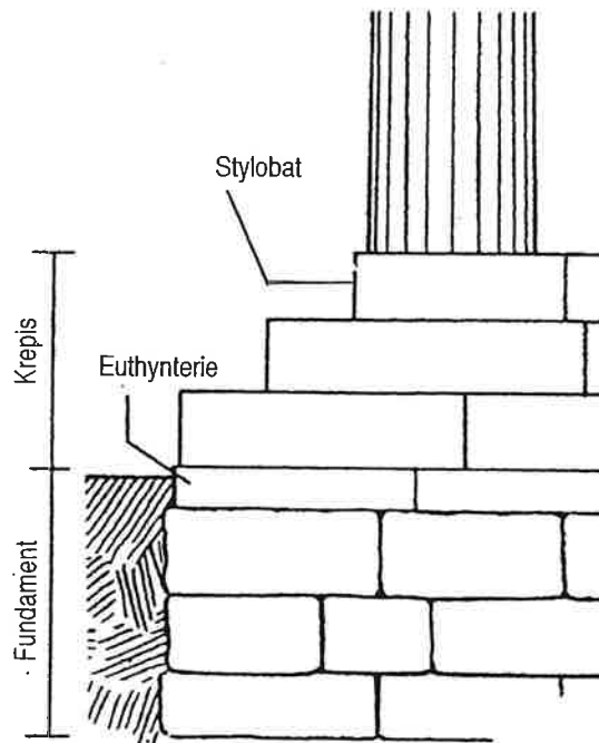
Die dorische Bauordnung: Säulenbasis
