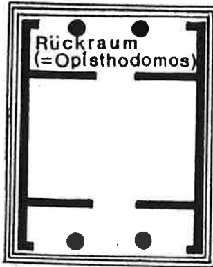
Doppelantentempel
