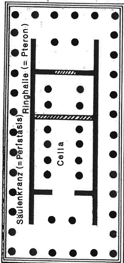
Apollontempel in Korinth (DORISCH)
