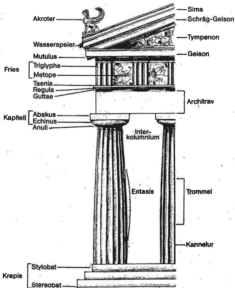
Fig. 1, Aufriß eines Tempels (vgl. auch S. 23)
