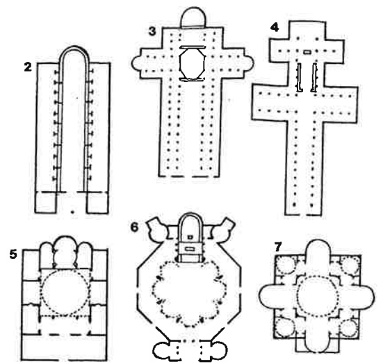
Fig. 2, Kirchentypen: 1 Idealgrundriß einer Basilika ohne Querschiff 2 Typus einer frühen Basilika (ab 4. Jh.) 3 lateinisches Kreuz (ab 6. Jh.) 4 Doppelkreuz (11. Jh.) 5, 6 Typen von Zentralbauten 7 griechisches Kreuz oder Kreuzkuppelkirchen
