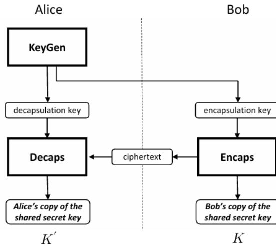
Figura 6.1: Funcionamiento del mecanismo KEM[25]
