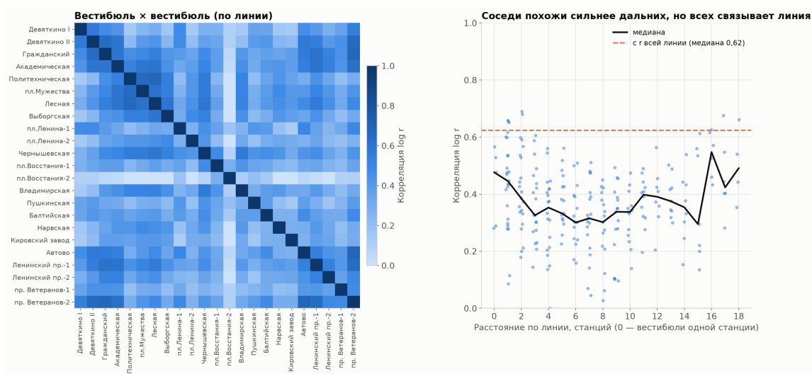
Рисунок 4.18 – СПб: корреляция отклонений между вестибюлями и с линией
