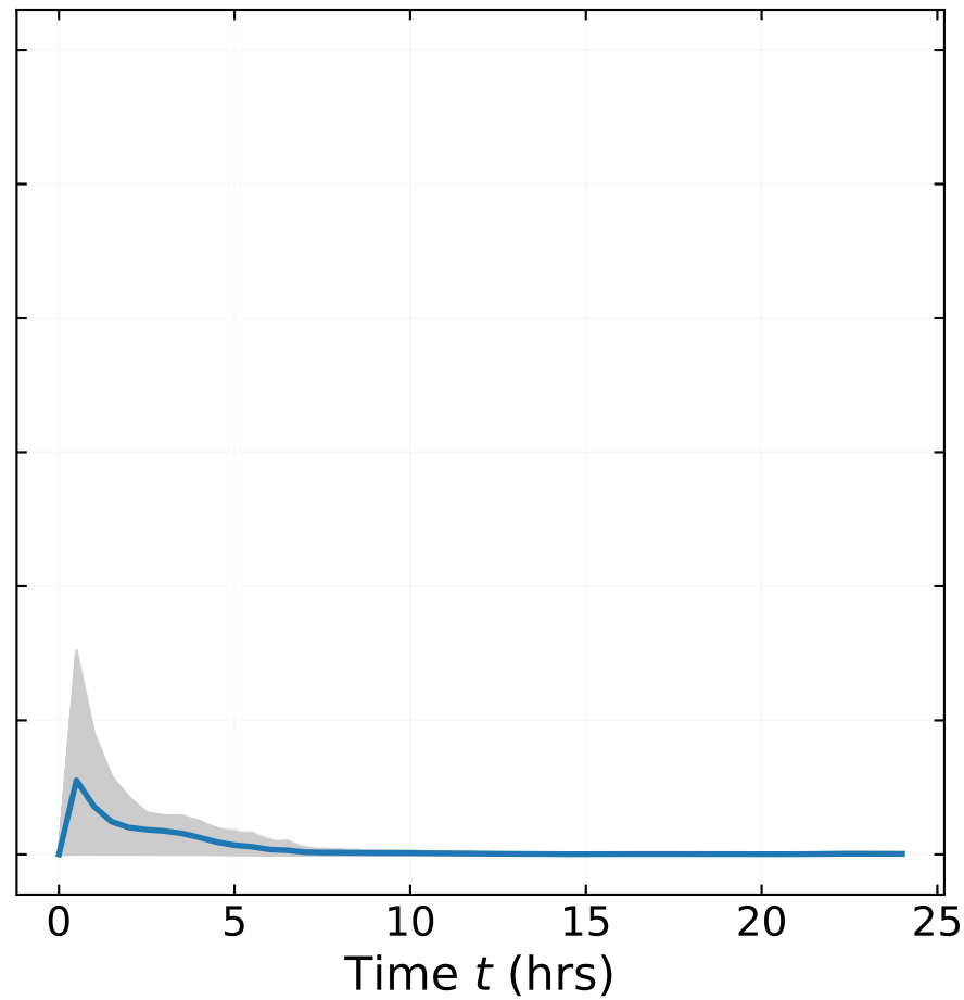
Untrained
