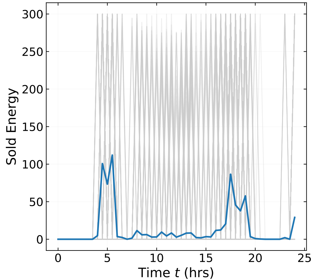
Heuristic
