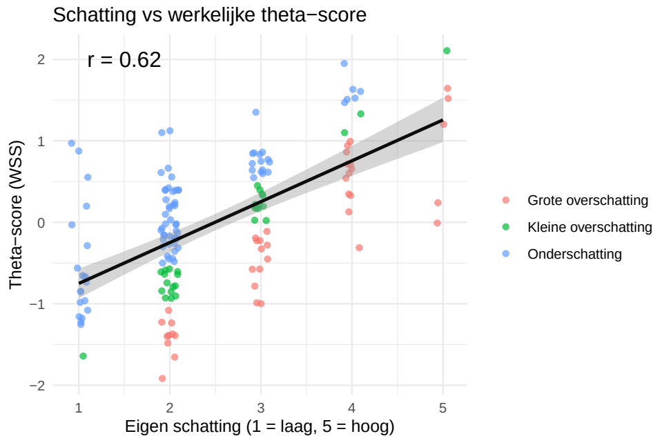
Figure 12: Scatterplot met trendlijn die de verhouding tussen schatting respondent en werkelijke score respondent weergeeft. Geannoteerd met kleuren die de mate van onder-/overschatting weergeven.
