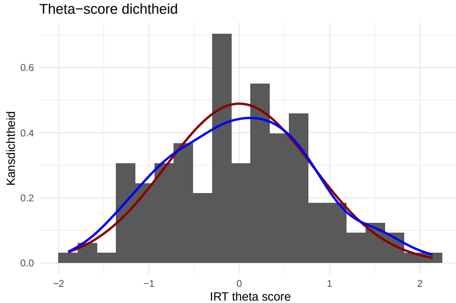
Figure 3: Geeft de kansdichtheid van de IRT-scores weer op basis van de behaalde scores. Met dichtheidscurve (blauw) en normaalcurve (rood)
