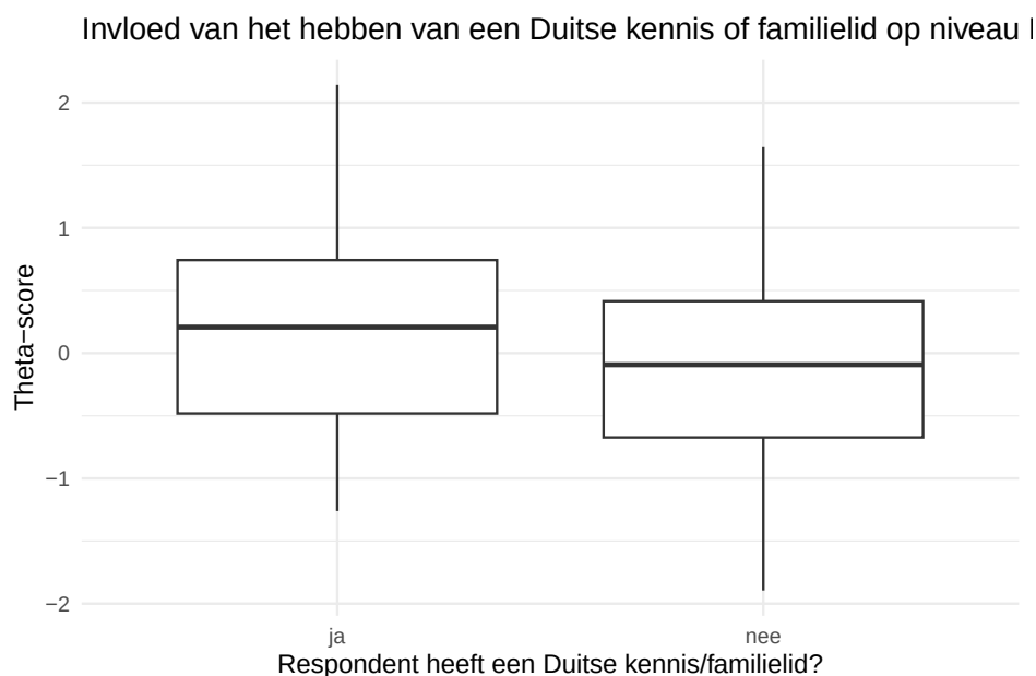
Figure 8: Een boxplot die de verdeling van theta-scores weergeeft van respondenten die wel/niet een Duitse kennis/familielid hebben.
