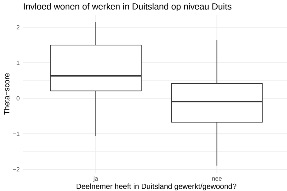
Figure 7: Een boxplot die de verdeling van theta-scores laat zien van respondenten die wel/niet in Duitsland hebben gewoond of gewerkt
