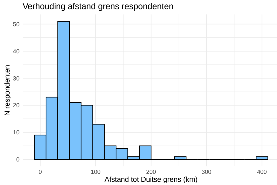
Figure 1: Verhouding afstand van Duitse grens tussen respondenten
