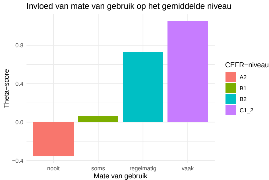
Figure 9: Barplot die de gemiddelde score per mate van gebruik weergeeft. Met geannoteerde kleur als CEFR-niveau.
