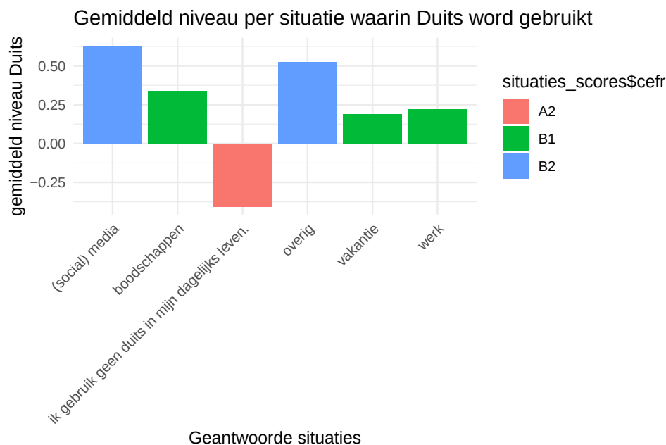
Figure 10: Barplot die de gemiddelde score per Duits-gebruikssituatie weergeeft. Met geannoteerde kleur als CEFR-niveau.
