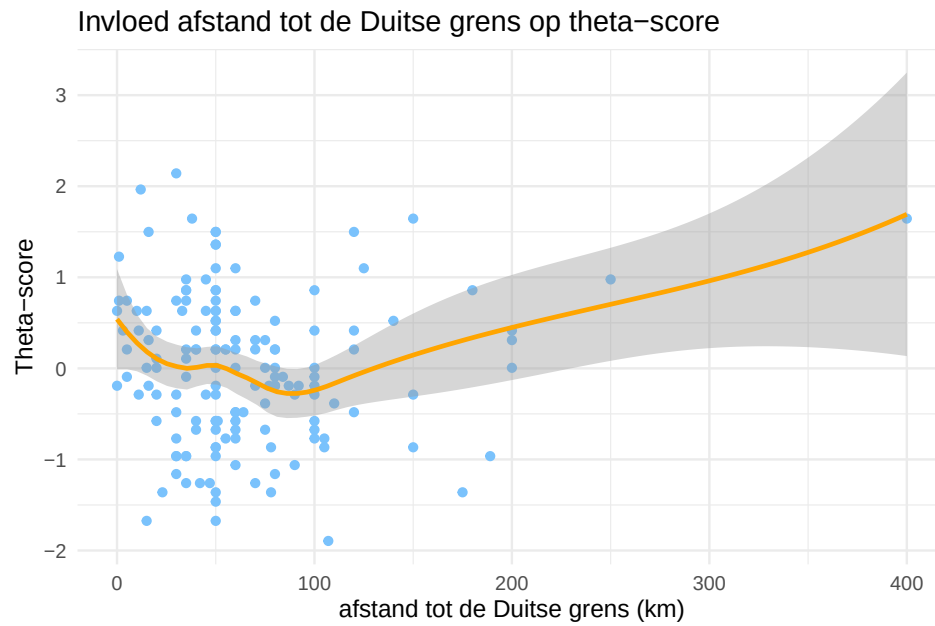
Figure 5: Scatter plot met een trendlijn (loess) dat de scores vergeleken met de afstand tot de grens weergeeft.
