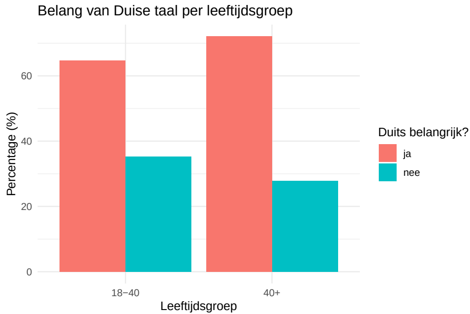
Figure 11: Percentage respondententen per leeftijdsgroep naar oordeel over het belang van de Duitse taal
