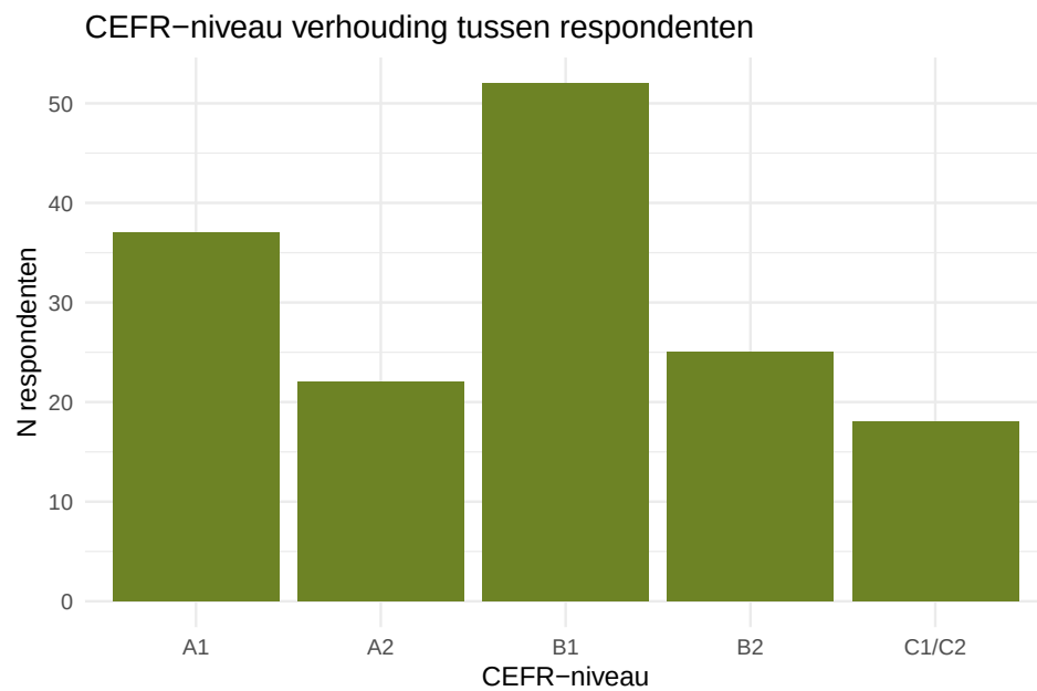
Figure 2: Laat zien hoeveel mensen elk CEFR-niveau beheersen.
