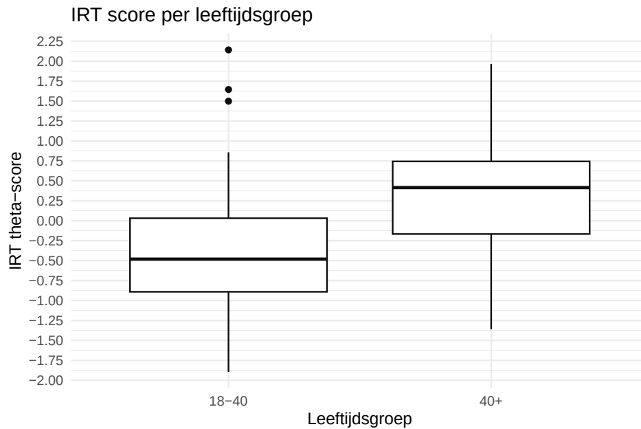
Figure 4: Boxplot dat de verdeling tussen leeftijdsgroepen en IRT-score weergeeft.
