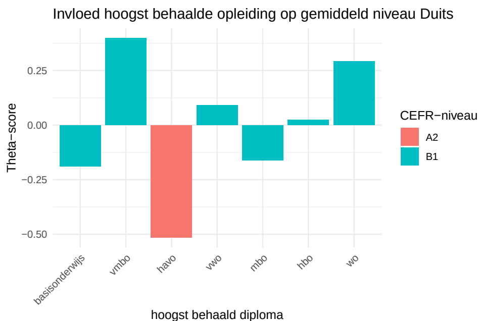
Figure 6: Een barplot die de gemiddelde CEFR-niveaus en theta-scores per hoogstbehaalde opleidingsniveau laat zien.
