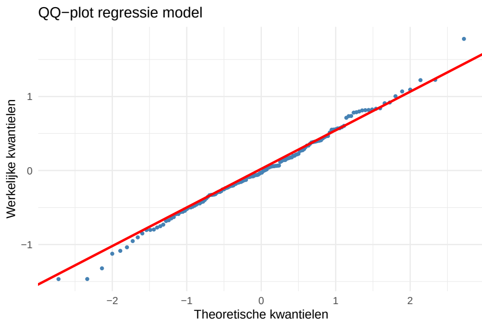
Figure 13: QQ-plot van de residuen ter beoordeling van de normaliteitsaannname. De S-vormige afwijking ten opzichte van de referentielijn wijst op een gestructureerd patroon in de residuen, wat suggereert dat het model de relatie met Duitse taalvaardigheid niet volledig lineair beschrijft.
