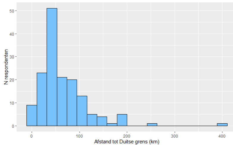
Figure 1: Verhouding afstand van Duitse grens tussen respondenten.
