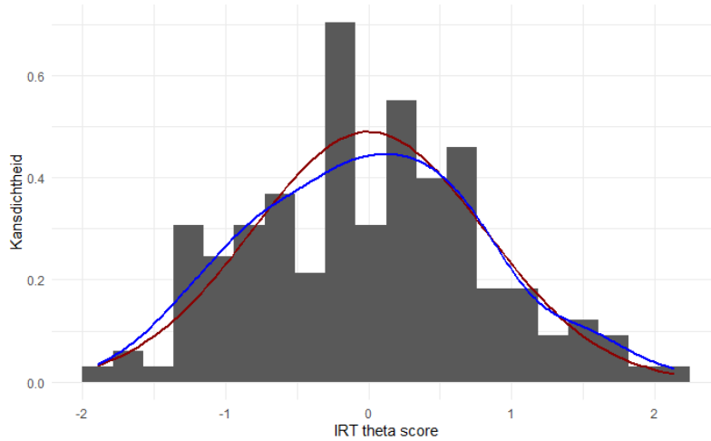
Figure 3: Theta-score dichtheid met dichtheidscurve (blauw) en normaalcurve (rood)
