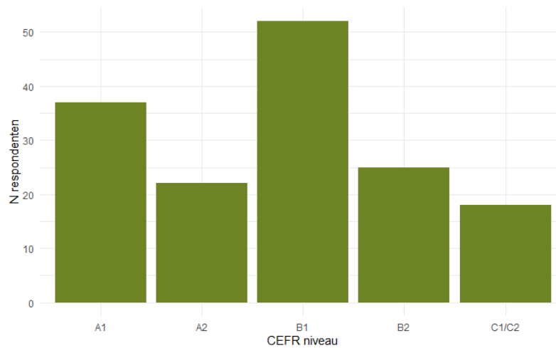
Figure 2: CEFR niveau verhouding tussen respondenten.
