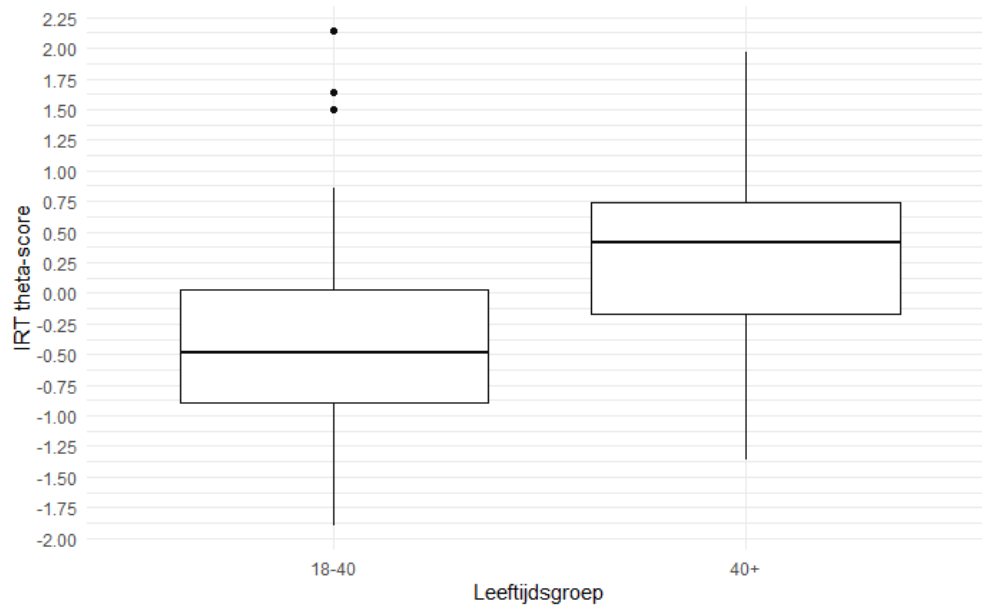
Figure 5: IRT score per leeftijdsgroep.
