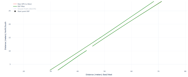
Figuur 36: Door het EKF aangevulde route (situatie 2).
