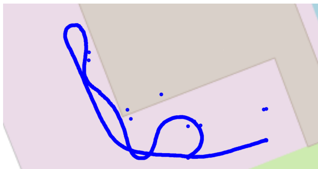
Figuur 21: Ruwe GNSS-route met softwarematig geïnjecteerde positiesprongen van 5 meter.
