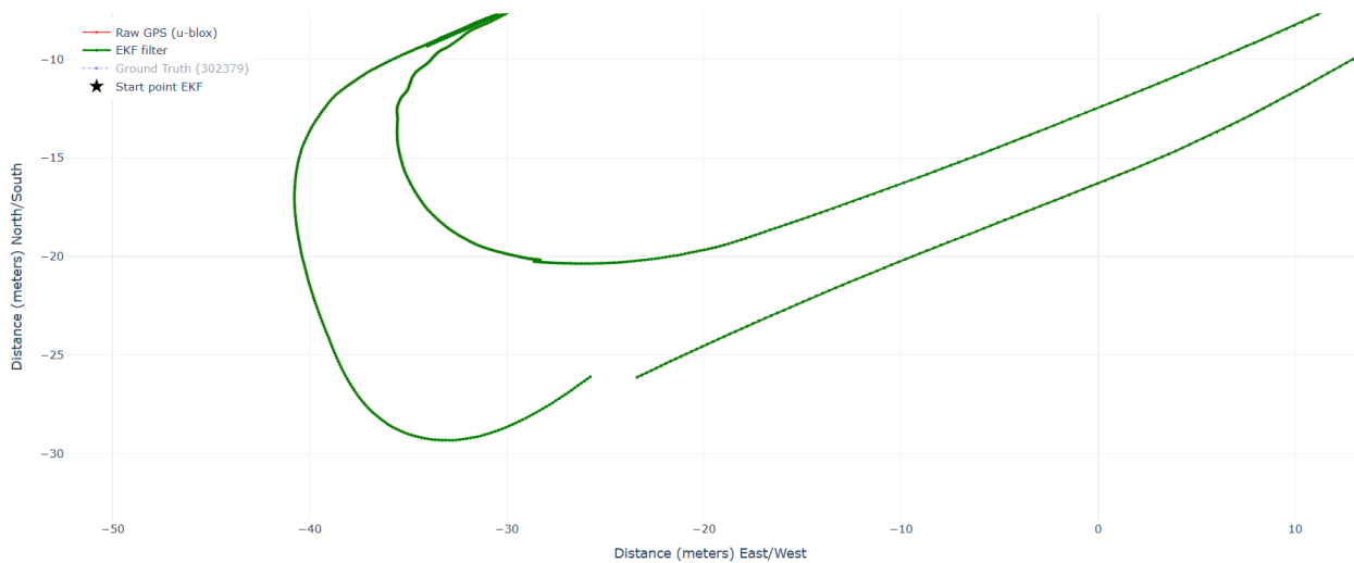
Figuur 34: Het EKF overbruggt de gaten, waarbij het onderste gat een lichte afwijking vertoont.
