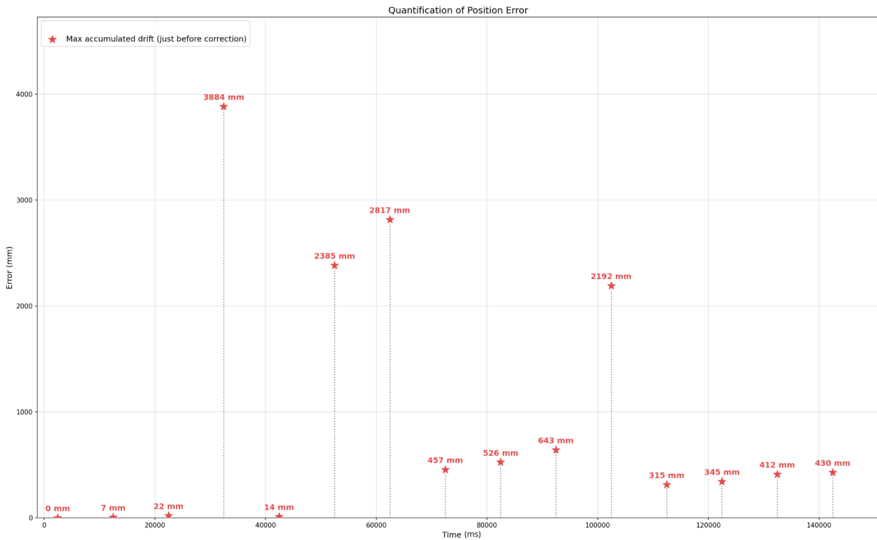
Figuur 39: Maximale opgebouwde positie afwijking van het EKF ten opzichte van de ruwe RTK positie, gemeten vlak vóór elke correctie na een signaaluitval. Deze afwijkingen zijn representatief voor de autotest. Elke ster vertegenwoordigt één uitval.
