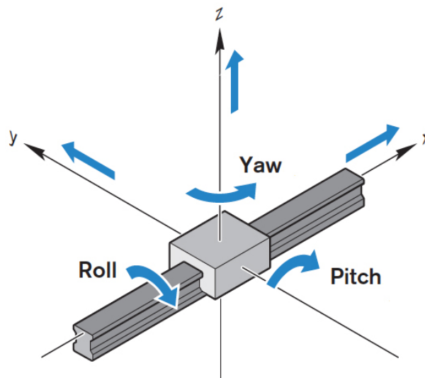
Figuur 6: De verschillende bewegingsdynamieken die een object ondervind zijn uitgedrukt in de pitch, roll en yaw [15].
