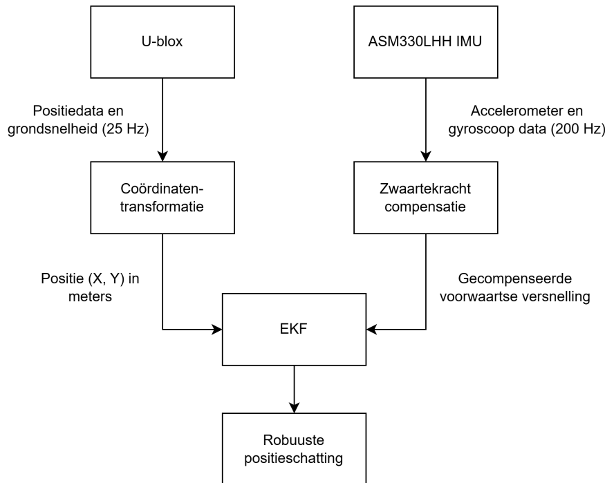
Figuur 11: In de afbeelding is de globale werking van het systeem schematisch weergegeven.
