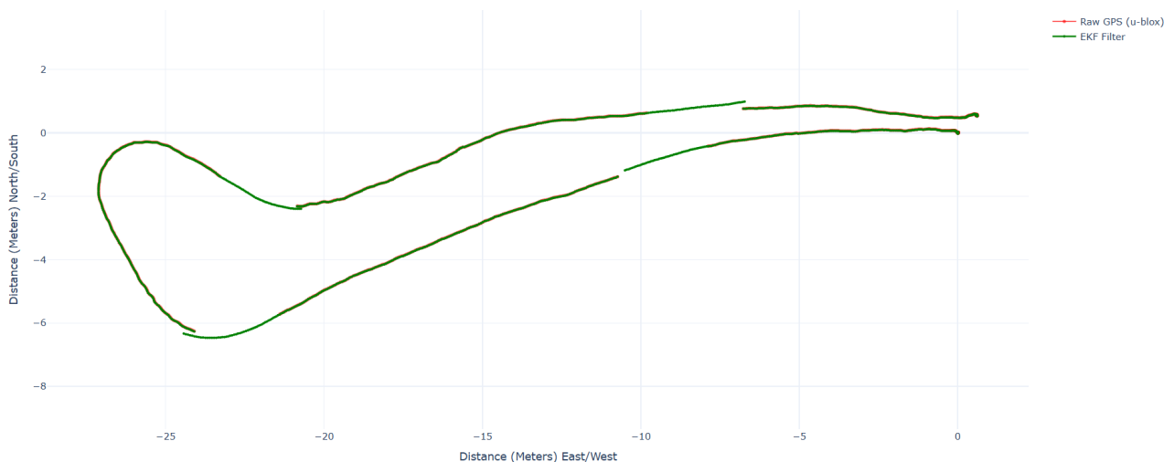
Figuur 31: Het EKF vult de gaten in het signaal op. Zichtbaar is een lichte positionele afwijking door drift.
