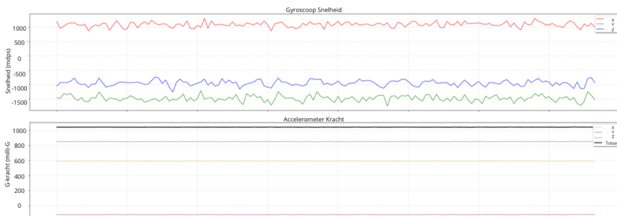
Figuur 14: Gyroscoop en accelerometer waardes bij stilstand op een tafel. Hierbij laat het bovenste venster de gyroscoop draaisnelheden zien en het onderste venster de g-krachten die de accelerometer waarneemt. De zwarte lijn is bedoeld om aan te tonen wat de totale g-kracht is die zich op het apparaat bevindt
