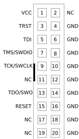
Figuur 13: Pinout van de JTAG connector waarbij pinnen 1, 7, 9 en GND zijn gebruikt voor de SWD-verbinding [19].
