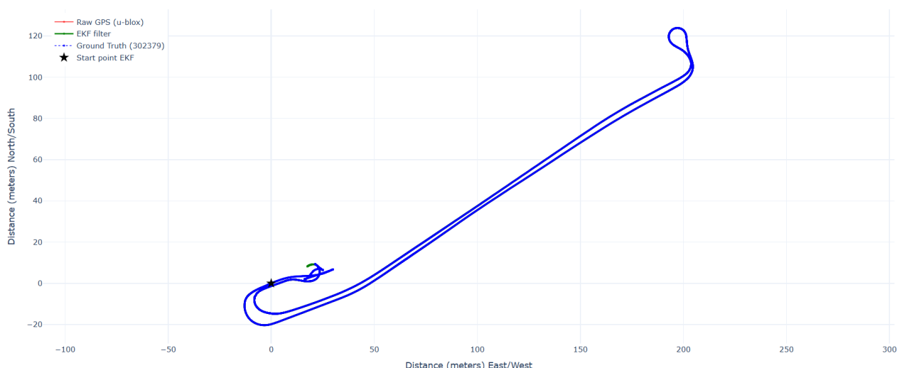
Figuur 20: Afgelegde route met de tracker gemonteerd op de auto. Het EKF blijft ook bij hogere snelheden nauwkeurig aansluiten op de RTK-positie.
