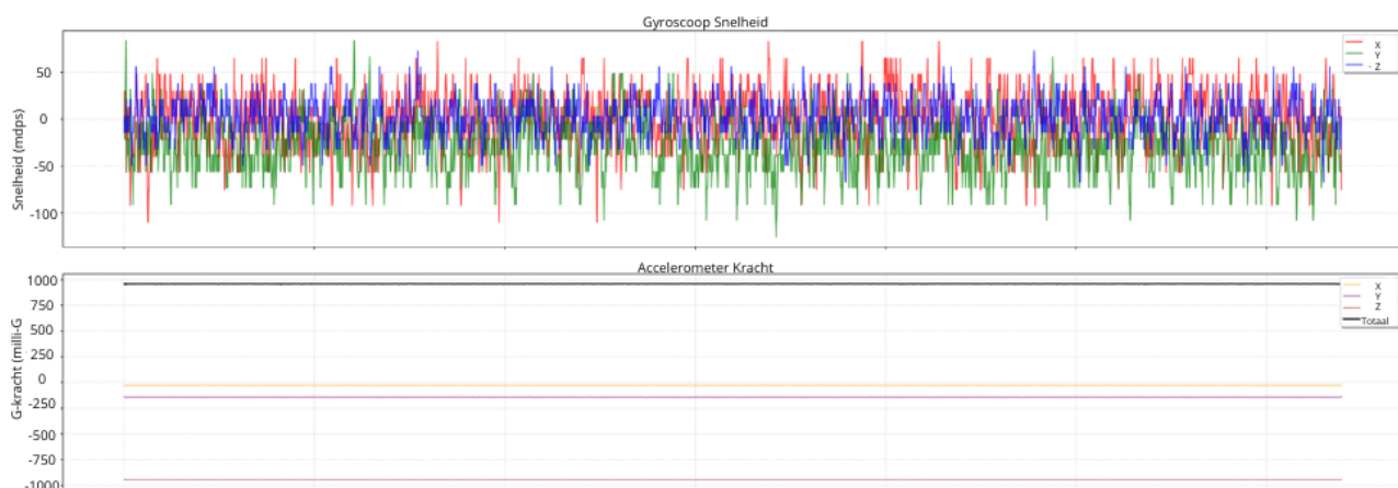
Figuur 16: De offset van de gyroscoop waardes zijn van de metingen afgetrokken
