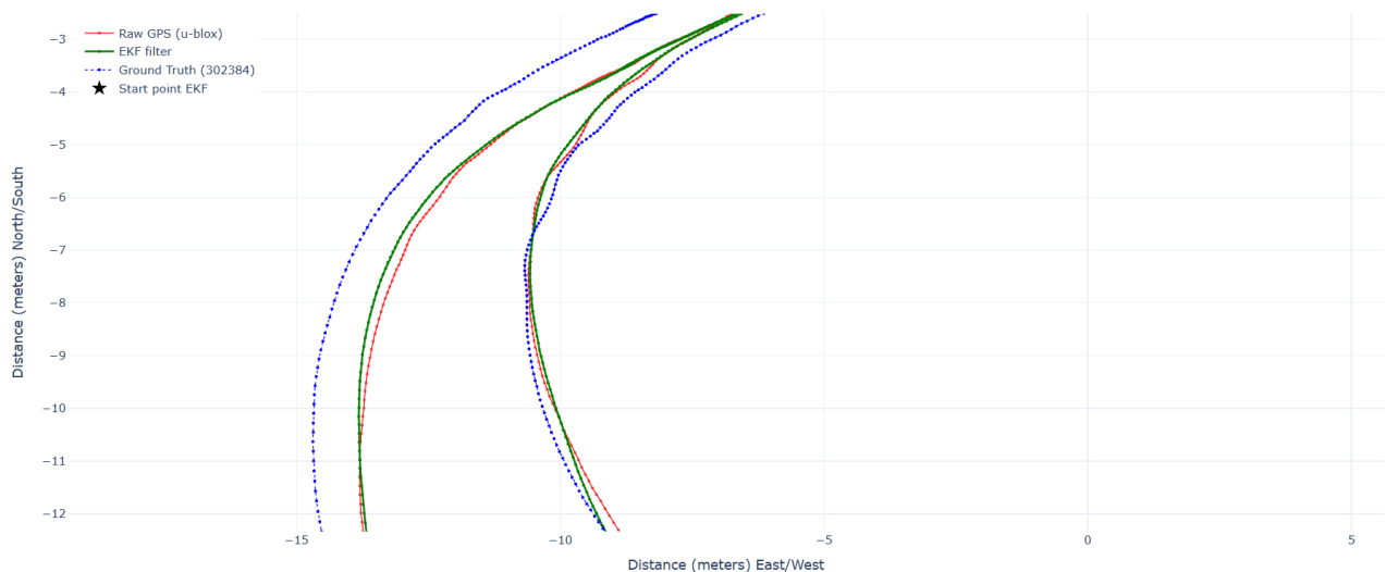
Figuur 29: Bocht tijdens de aanvullende autotest. De ruwe GNSS-positie toont een schommeling door een drempel; het EKF vlakt dit af naar een vloeiende boog doordat het model geen verticale bewegingen modelleert.
