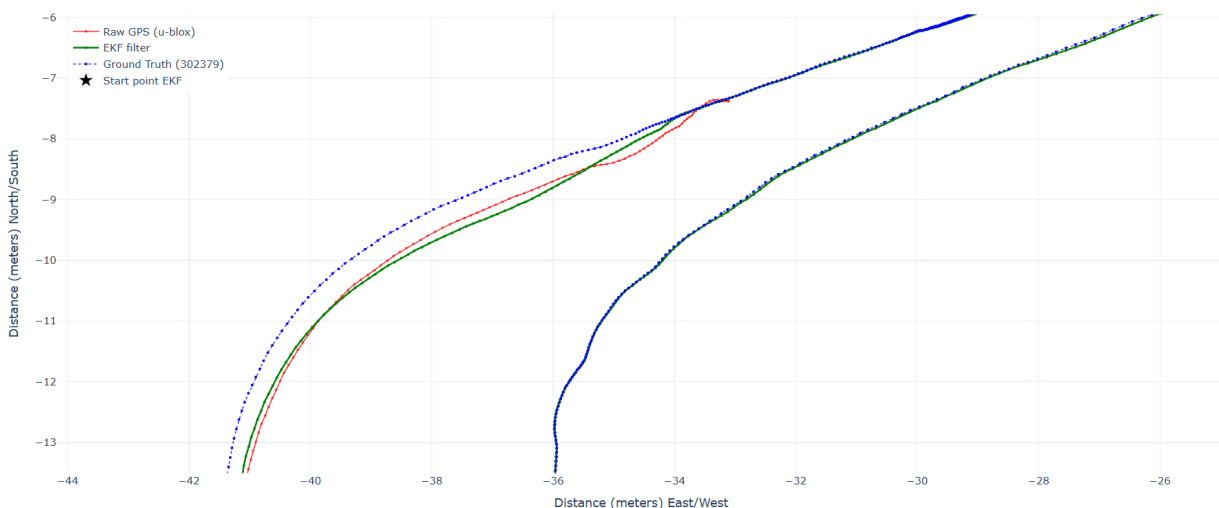
Figuur 27: Ingezoomd moment tijdens de autotest. Het EKF trekt de route kortdurend goed door maar drift langzamerhand mee met de foutieve positie.
