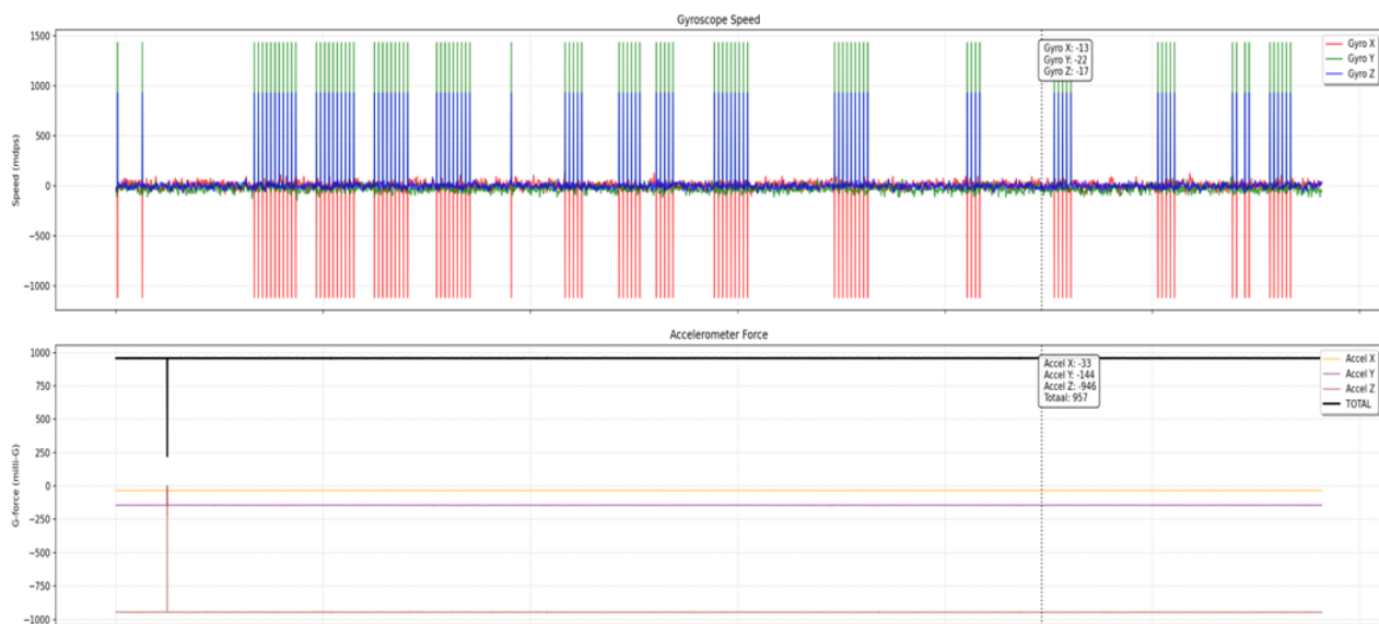
Figuur 17: Willekeurige grote pieken in de gyroscoop data. Dit zijn resultaten op een stilstaande tafel
