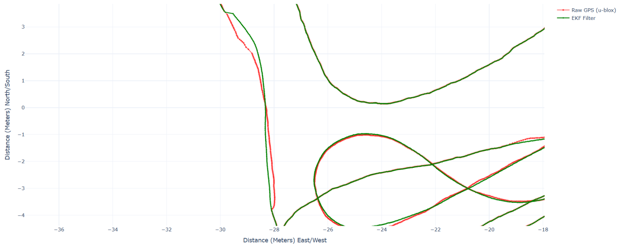
Figuur 25: Ingezoomd moment waarbij de ruwe GNSS-positie een plotselinge sprong maakt. Het EKF trekt de route logisch door maar drift na verloop van tijd mee met de foutieve positie.
