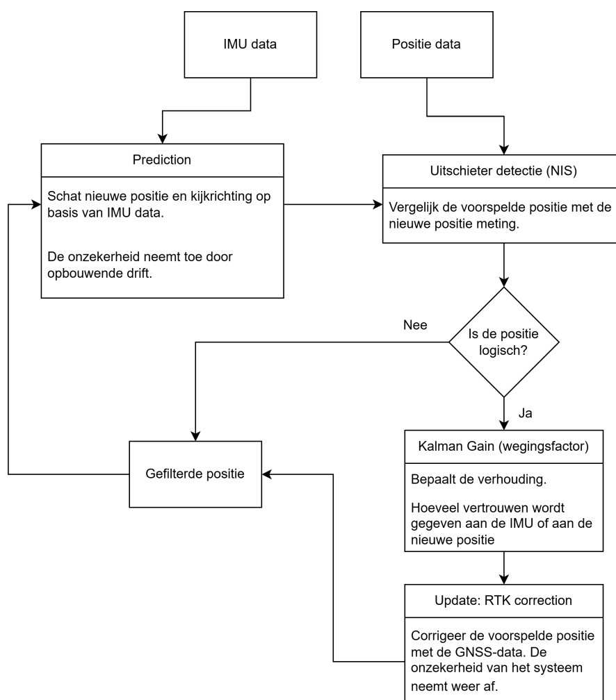
Figuur 12: In de afbeelding is de globale werking van het EKF uitgebeeld
