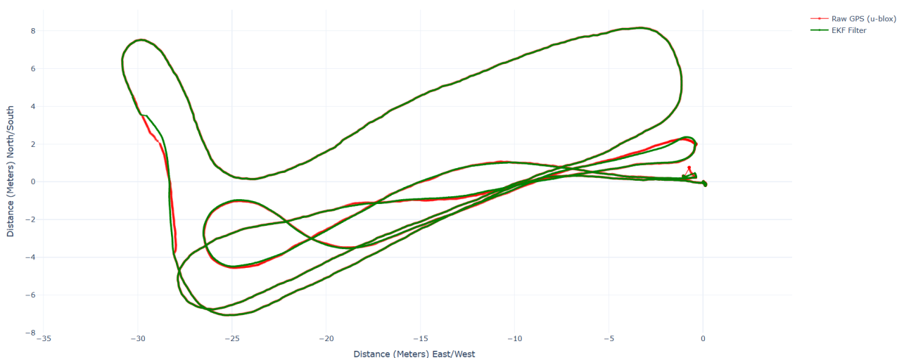
Figuur 24: Looproute met uitgeschakelde RTCM-correcties. Op meerdere momenten wijkt de EKF-positie af van de foutieve GNSS-positie.
