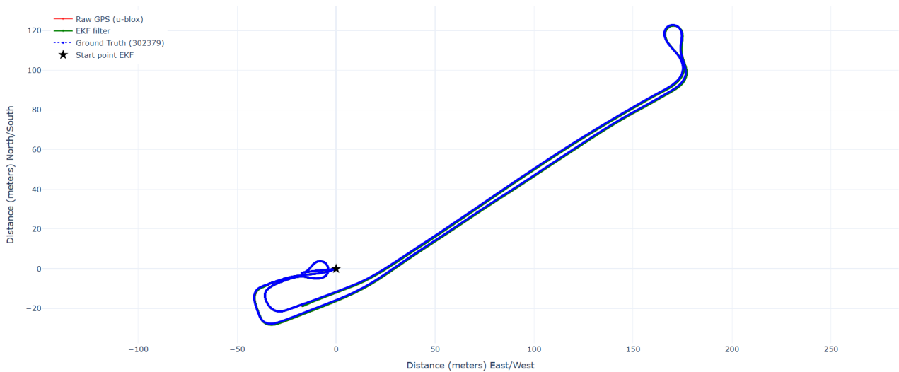
Figuur 26: Autoroute met uitgeschakelde RTCM-correcties. Het EKF wijkt op meerdere momenten af van de foutieve GNSS-positie.
