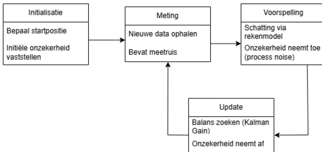
Figuur 4: In de afbeelding is de globale werking van een kalman filter schematisch weergegeven. Hierbij wordt de gehele cyclus elke tijdsstap doorlopen.
