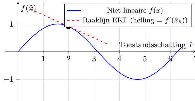
Figuur 5: Het kernprincipe van het Extended Kalman Filter in één dimensie. De niet-lineaire functie f(x) (blauw) wordt op elk tijdstip lokaal benaderd door een raaklijn (rood gestippeld) in het huidige schattingspunt \hat{x}_k . De helling van die raaklijn is gelijk aan de afgeleide f'(\hat{x}_k) . Het standaard Kalman Filter veronderstelt dat het systeem altijd globaal lineair is; het EKF herberekent deze lokale benadering bij elke tijdstap opnieuw [2].
