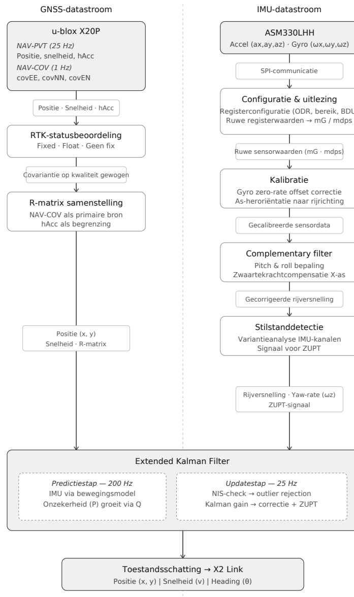
Figuur 7: Blokschema waarin de systeemarchitectuur uitgebeeld is. De twee datastromen worden voorverwerkt voordat zij de EKF bereiken.
