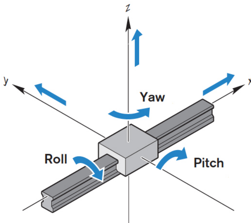
Figuur 3: De verschillende bewegingsdynamieken die een object ondervindt zijn uitgedrukt in de pitch, roll en yaw [12].
