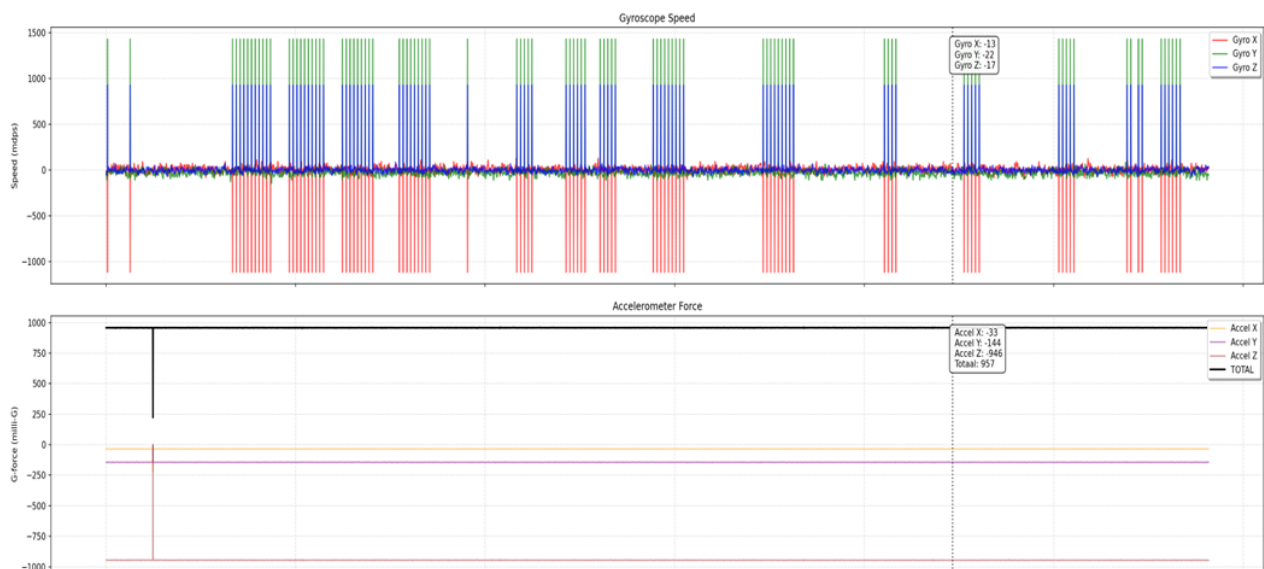
Figuur 14: Willekeurige grote pieken in de gyroscoop data. Dit zijn resultaten op een stilstaande tafel
