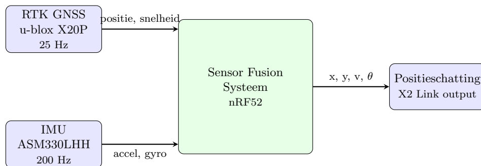
Figuur 6: Blackbox overzicht het sensor fusion systeem ontvangt twee asynchrone datastromen en levert één betrouwbare positieschatting. Deze wordt vervolgens door het X2-Link protocol verstuurd.
