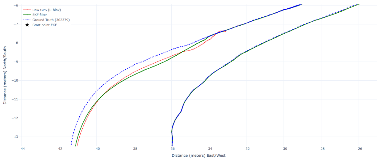
Figuur 25: Ingezoomd moment tijdens de autotest. Het EKF trekt de route kortdurend goed door maar drift langzamerhand mee met de foutieve positie.
