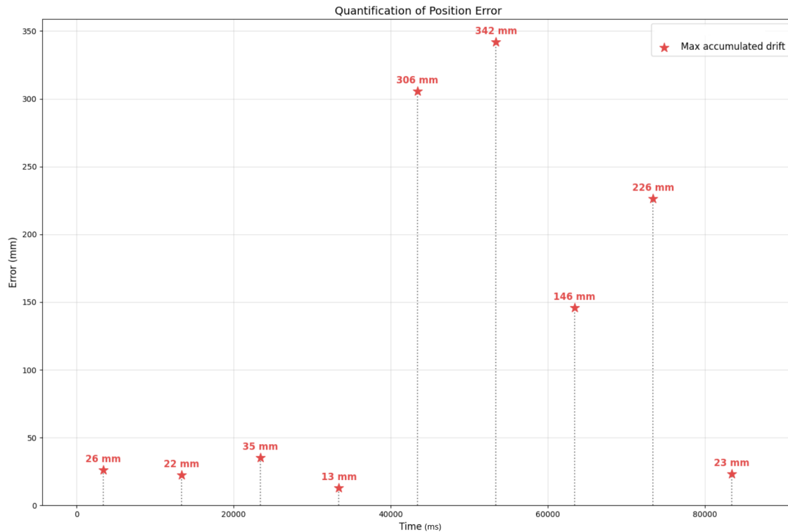
Figuur 30: Maximale opgebouwde positie afwijking van het EKF ten opzichte van de ruwe RTK positie, gemeten vlak vóór elke correctie na een signaaluitval. Deze afwijkingen zijn representatief voor de looptest. Elke ster vertegenwoordigt één uitval.
