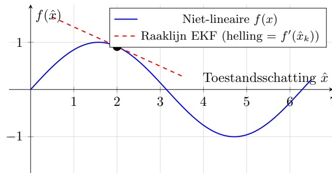
Figuur 6: Het kernprincipe van het Extended Kalman Filter in één dimensie. De niet-lineaire functie f(x) (blauw) wordt op elk tijdstip lokaal benaderd door een raaklijn (rood gestippeld) in het huidige schattingspunt \hat{x}_k . De helling van die raaklijn is gelijk aan de afgeleide f'(\hat{x}_k) . Het standaard Kalman Filter veronderstelt dat het systeem altijd globaal lineair is; het EKF herberekent deze lokale benadering bij elke tijdstap opnieuw [2].
