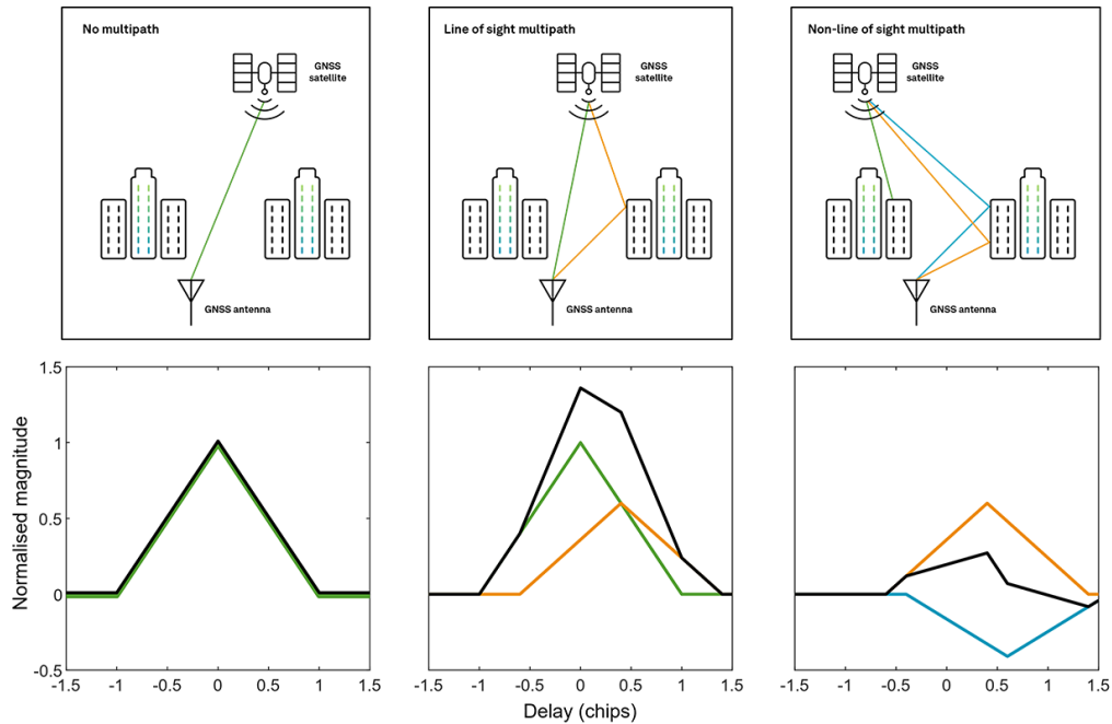
Figuur 3: In de afbeelding is het effect van zowel multipath als non line of sight in statistieken uiteengezet. De groene lijn staat voor het directe signaal, en de gele en blauwe staan voor de multipath signalen. De zwarte lijn is wat de ontvanger waarneemt [20]
