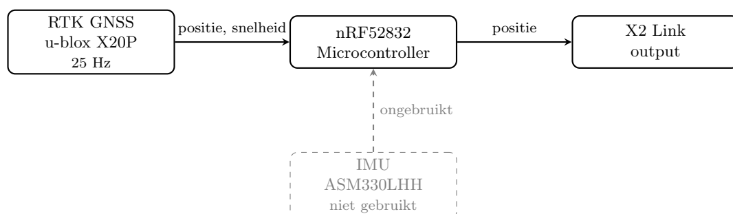
Figuur 1: Werking van het huidige systeem. De positiebepaling is volledig gebaseerd op de RTK GNSS-ontvanger. De IMU is fysiek aanwezig maar wordt niet ingezet voor de positiebepaling.
