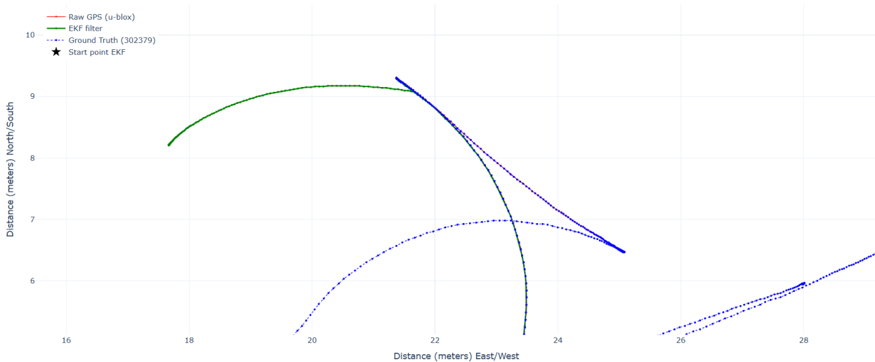
Figuur 21: Achteruitrijden tijdens de autotest. De EKF positie beweegt vooruit omdat de u-blox receiver geen rijrichting meelevert en het model geen achteruitrijden opvangt.
