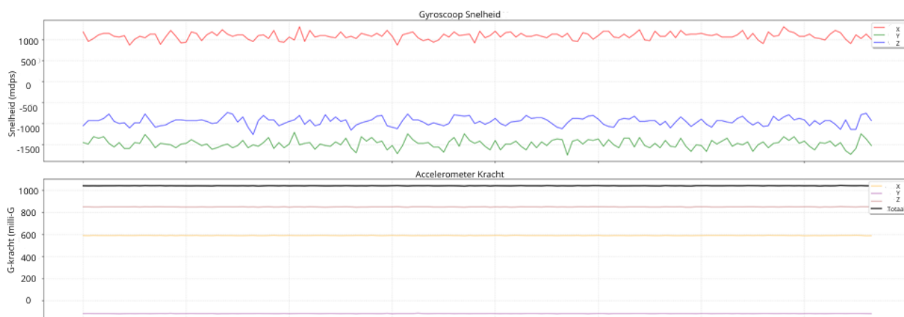
Figuur 12: Gyroscoop en accelerometer waardes bij stilstand op een tafel. Hierbij laat het bovenste venster de gyroscoop draaisnelheden zien en het onderste venster de g-krachten die de accelerometer waarneemt. De zwarte lijn is bedoeld om aan te tonen wat de totale g-kracht is die zich op het apparaat bevindt
