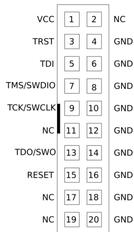
Figuur 11: Pinout van de JTAG connector waarbij pinnen 1, 7, 9 en GND zijn gebruikt voor de SWD-verbinding [16].
