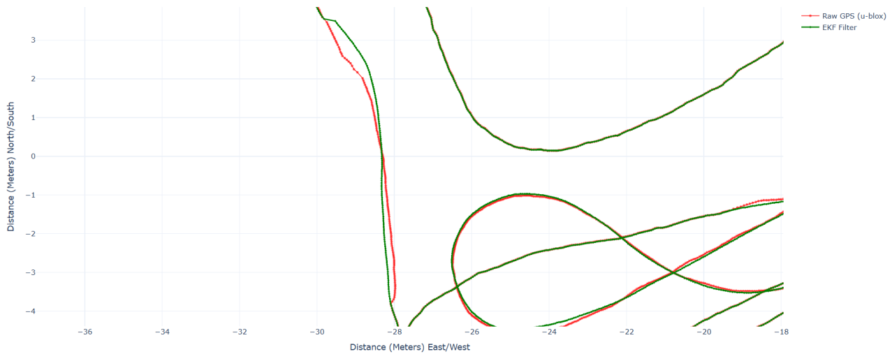
Figuur 23: Ingezoomd moment waarbij de ruwe GNSS-positie een plotselinge sprong maakt. Het EKF trekt de route logisch door maar driftt na verloop van tijd mee met de foutieve positie.
