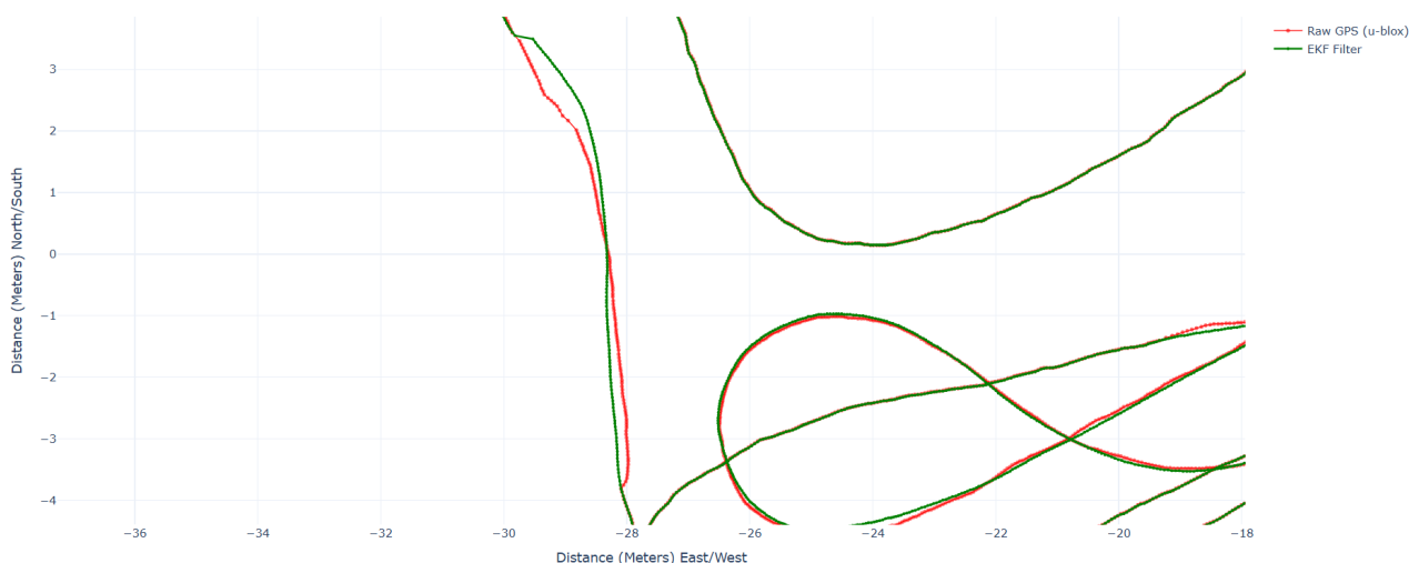
Figuur 25: Ingezoomd moment waarbij de ruwe GNSS-positie een plotselinge sprong maakt. Het EKF trekt de route logisch door maar drift na verloop van tijd mee met de foutieve positie.
