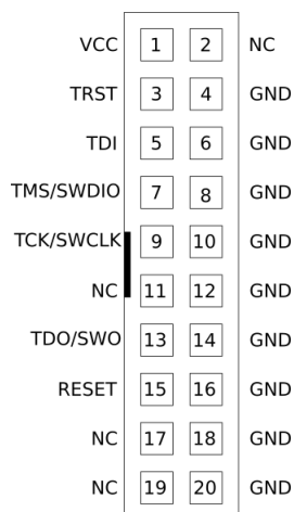
Figuur 13: Pinout van de JTAG connector waarbij pinnen 1, 7, 9 en GND zijn gebruikt voor de SWD-verbinding [21].
