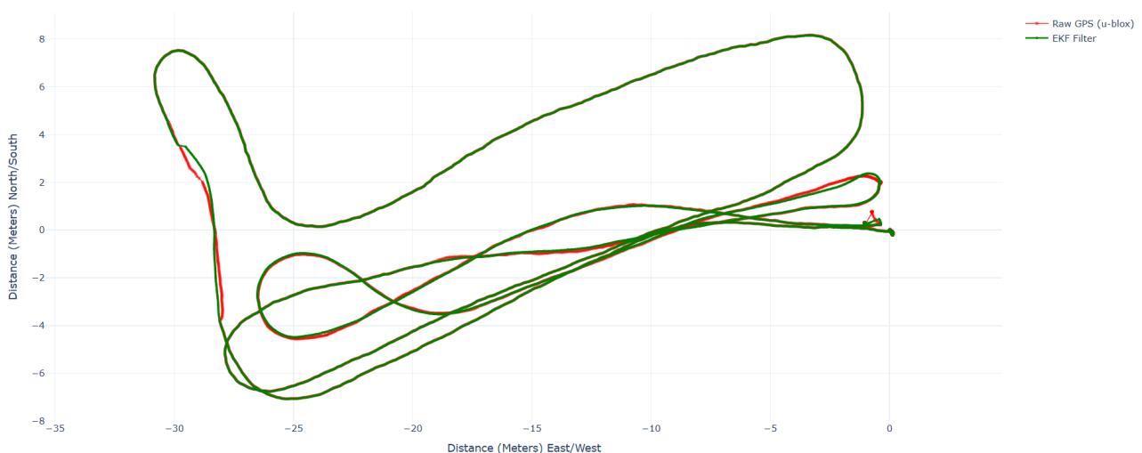
Figuur 24: Looproute met uitgeschakelde RTCM-correcties. Op meerdere momenten wijkt de EKF-positie af van de foutieve GNSS-positie.
