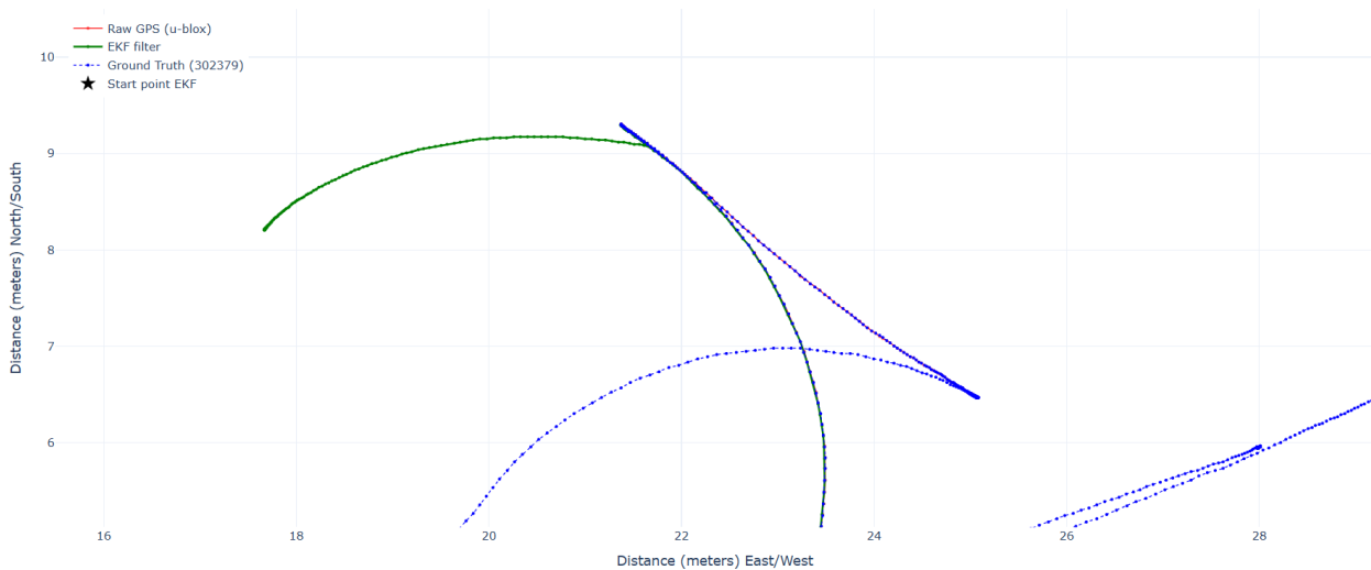
Figuur 23: Achteruitrijden tijdens de autotest. De EKF positie beweegt vooruit omdat de u-blox receiver geen rijrichting meeleeft en het model geen achteruitrijden opvangt.
