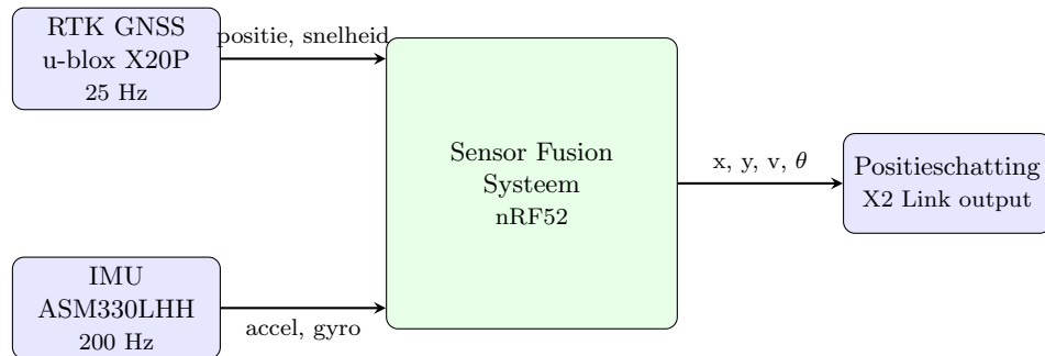
Figuur 7: Blackbox overzicht het sensor fusion systeem ontvangt twee asynchrone datastromen en levert één betrouwbare positieschatting. Deze wordt vervolgens door het X2-Link protocol verstuurd.
