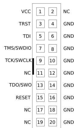
Figuur 8: Pinout van de JTAG connector [15]
