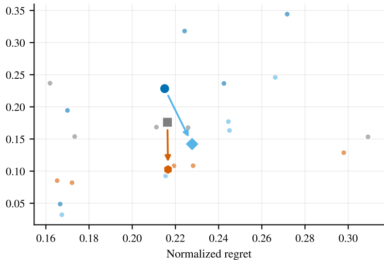
Multidimensional knapsack
