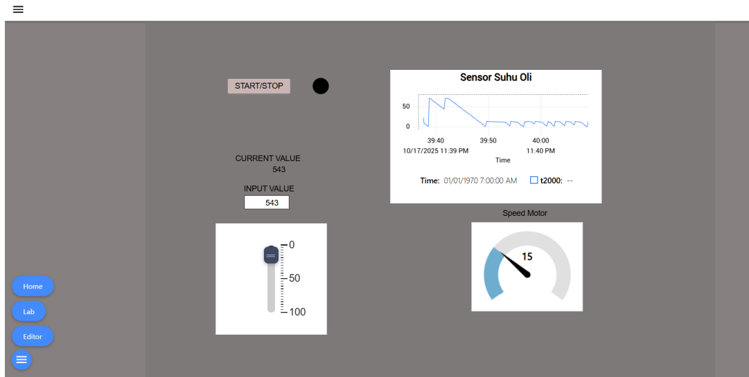
Gambar 4.8: Demo sistem HMI saat berjalan dan berkomunikasi langsung dengan PLC secara realtime. Antarmuka menampilkan visualisasi data berupa grafik (chart) dan kontrol input berupa slider yang responsif terhadap nilai aktual di PLC.
