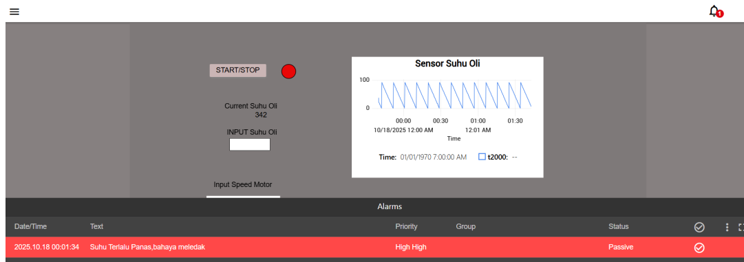
Gambar 4.9: Tampilan demo alarm pada HMI ketika suhu oli melebihi batas aman. Sistem menampilkan notifikasi visual dengan tingkat prioritas High High.
