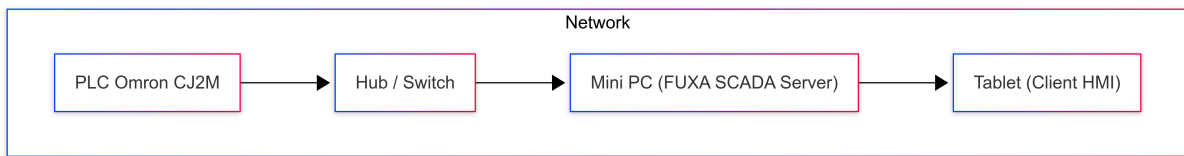
Gambar 3.2: Topologi Sistem SCADA FUXA dengan Protokol FINS (Mini PC, PLC, Hub, Tablet)
