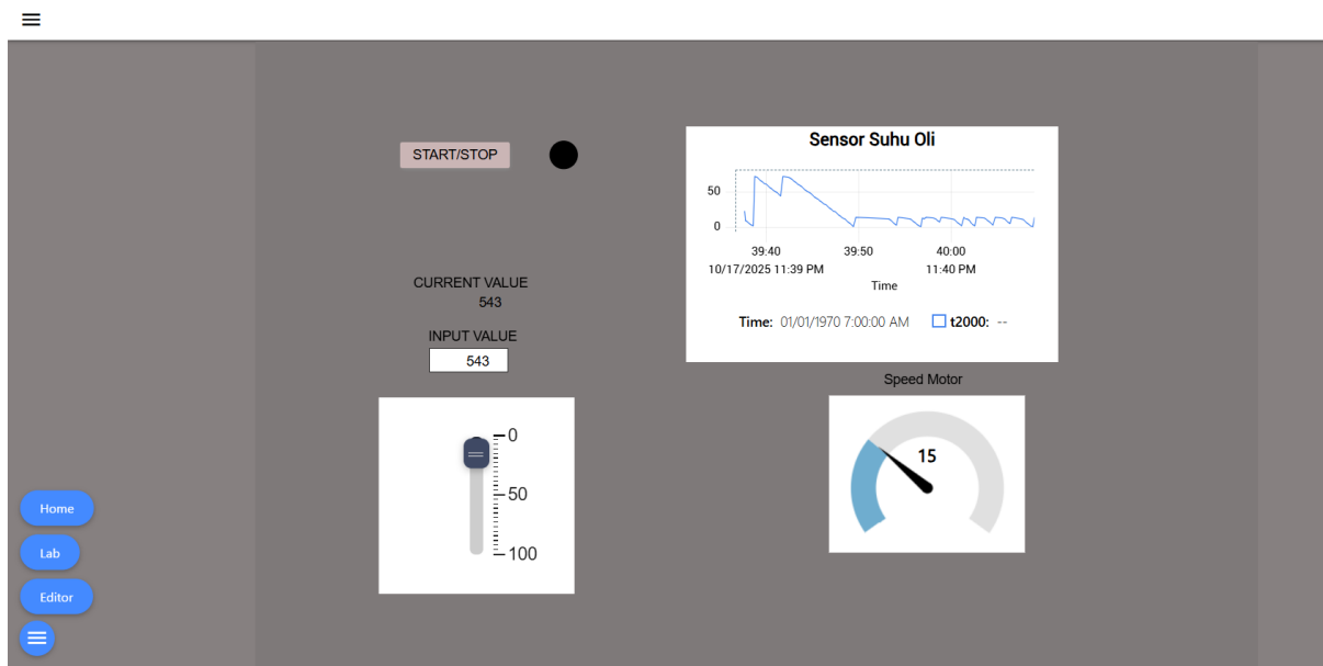
Gambar 4.9: Demo sistem HMI yang terkoneksi dengan PLC secara real-time. Antarmuka menampilkan visualisasi data berupa grafik (chart) dan kontrol input berupa slider yang responsif terhadap nilai aktual di PLC.
