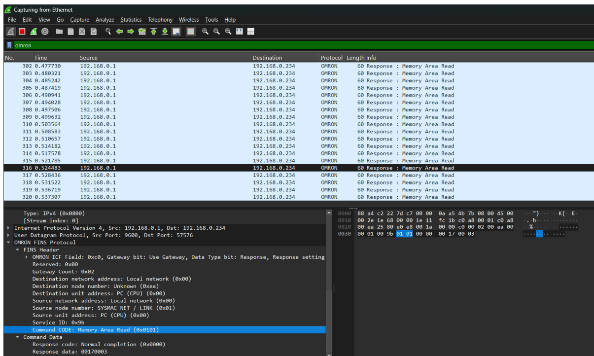
Gambar 4.4: Cuplikan hasil analisis paket FINS pada Wireshark
