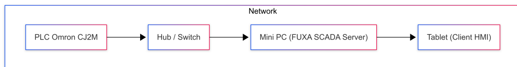
Gambar 4.5: Topologi sistem HMI FUXA dengan konektor FINS
