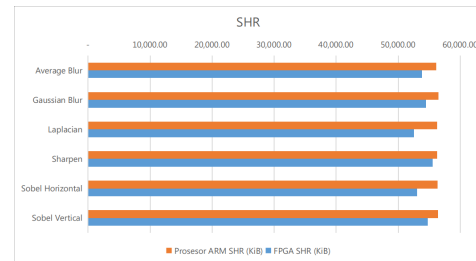
Gambar 17: Grafik perbandingan penggunaan shared memory (SHR) dengan menggunakan prosesor ARM dan FPGA.
