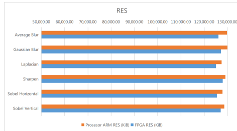
Gambar 16: Grafik perbandingan penggunaan resident memory (RES) dengan menggunakan prosesor ARM dan FPGA.
