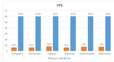
Gambar 13: Grafik perbandingan FPS dengan menggunakan prosesor ARM dan FPGA.
