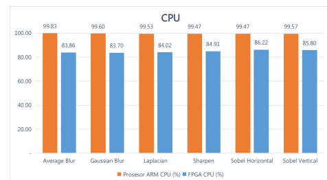
Gambar 14: Grafik perbandingan penggunaan CPU dengan menggunakan prosesor ARM dan FPGA.
