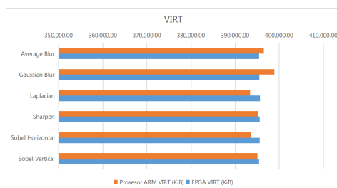
Gambar 18: Grafik perbandingan penggunaan virtual memory (VIRT) dengan menggunakan prosesor ARM dan FPGA.
