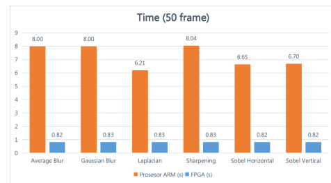
Gambar 11: Grafik perbandingan waktu komputasi dengan 50 frame dan 200 frame
