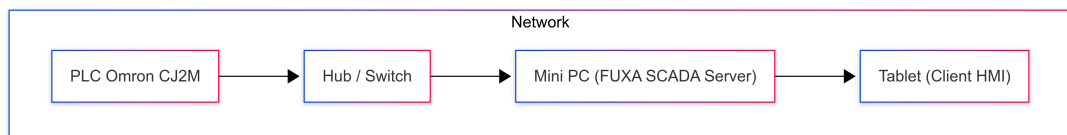
Gambar 3.2: Topologi Sistem SCADA FUXA dengan Protokol FINS (PC, PLC, Hub, Tablet)
