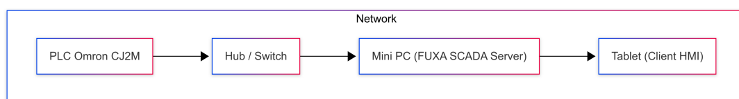
Gambar 4.4: Topologi sistem HMI FUXA dengan konektor FINS
