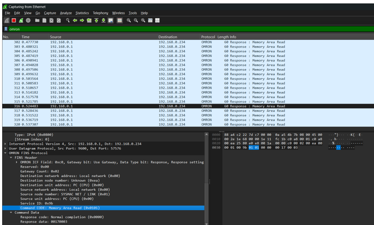
Gambar 4.3: Cuplikan hasil analisis paket FINS pada Wireshark
