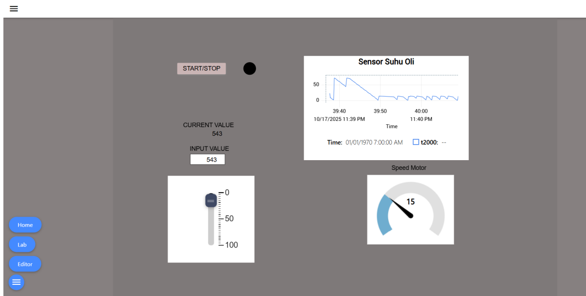
Gambar 4.8: Demo sistem HMI saat berjalan dan berkomunikasi langsung dengan PLC secara realtime . Antarmuka menampilkan visualisasi data berupa grafik ( chart ) dan kontrol input berupa slider yang responsif terhadap nilai aktual di PLC.
