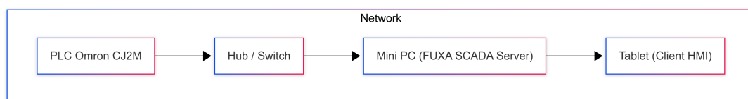
Gambar 4.5: Topologi sistem HMI FUXA dengan konektor FINS
