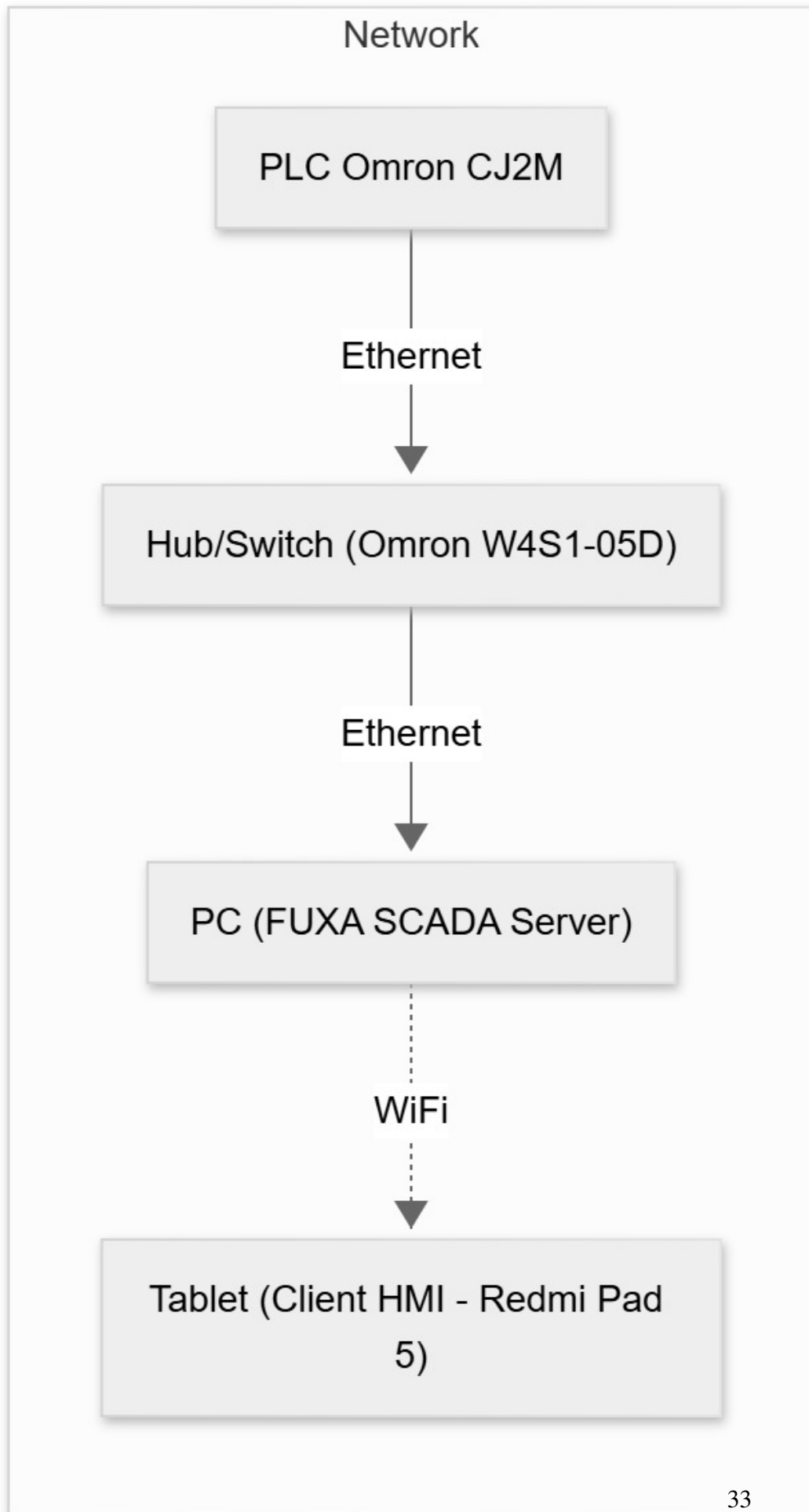
Gambar 4.5: Topologi sistem HMI FUXA dengan konektor FINS
