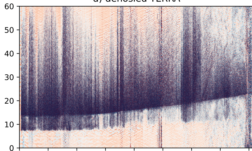
e) denosied TERRA: P-wave
