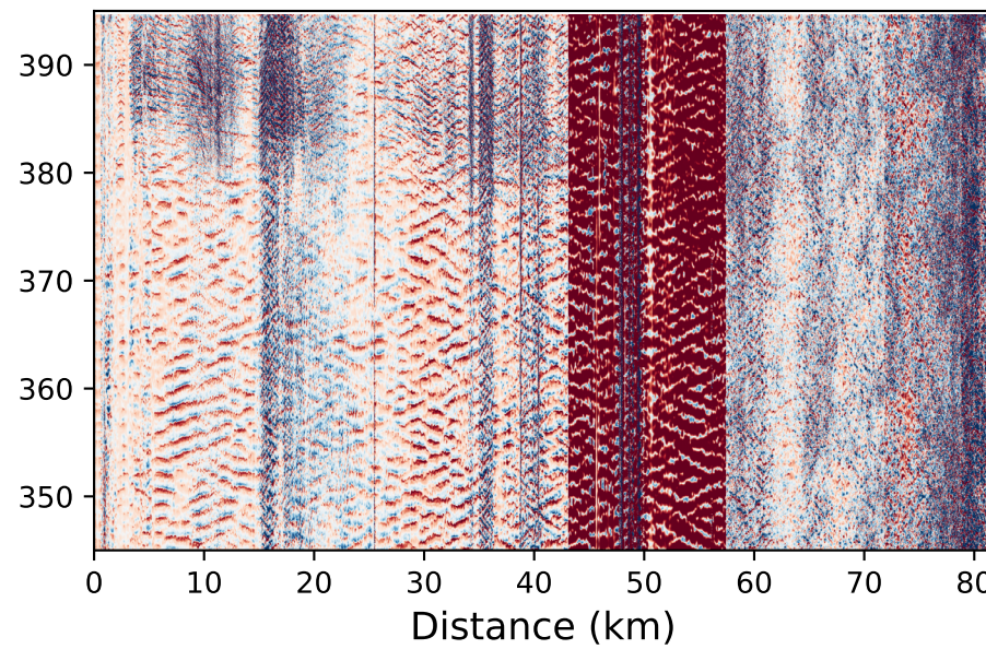
f) denosied TERRA: S-wave
