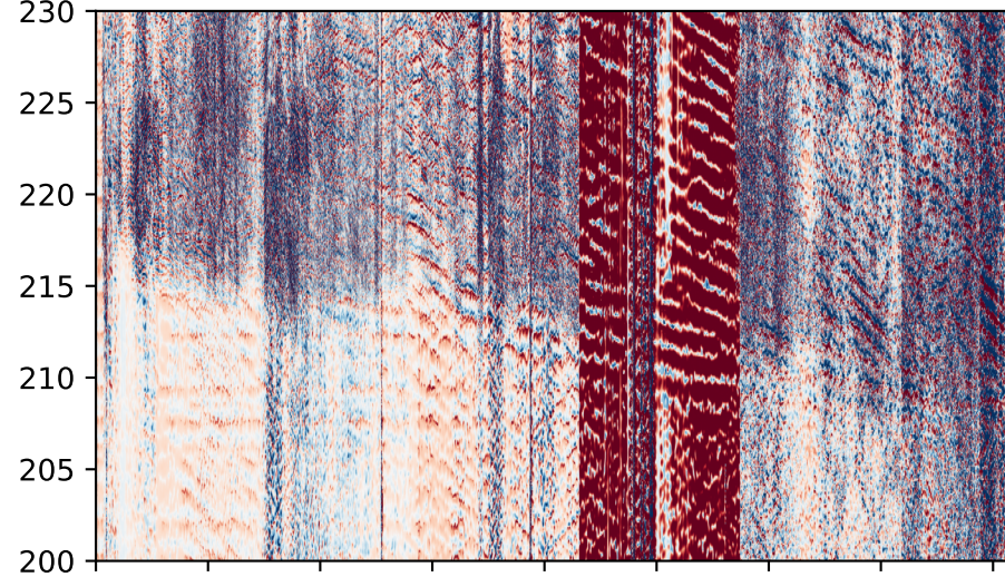
f) denosied TERRA: S-wave
