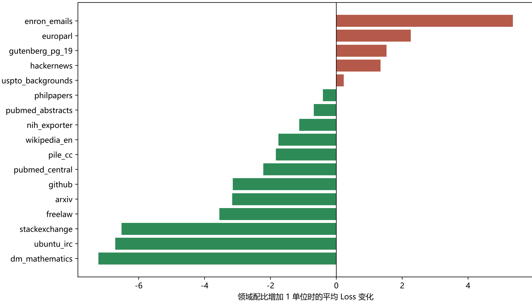
各预训练领域对平均 Loss 的局部边际效应
