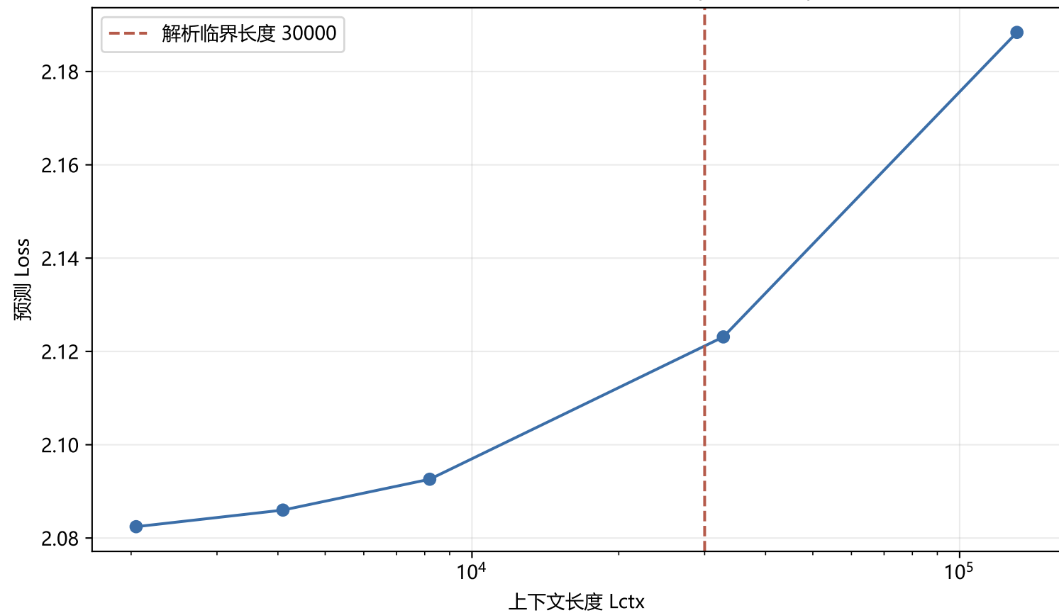
上下文长度对最优预测 Loss 的影响 ( C=1e+22 )
