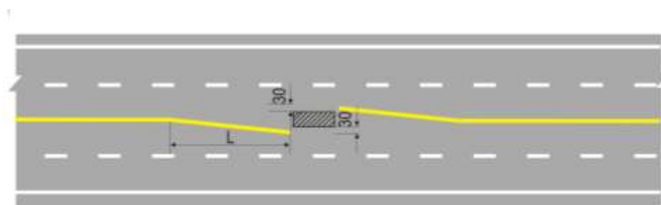
Hình G.25 - Bố trí vạch sơn cho đường có từ 4 làn xe trở lên khi có chướng ngại vật nằm ở giữa đường
