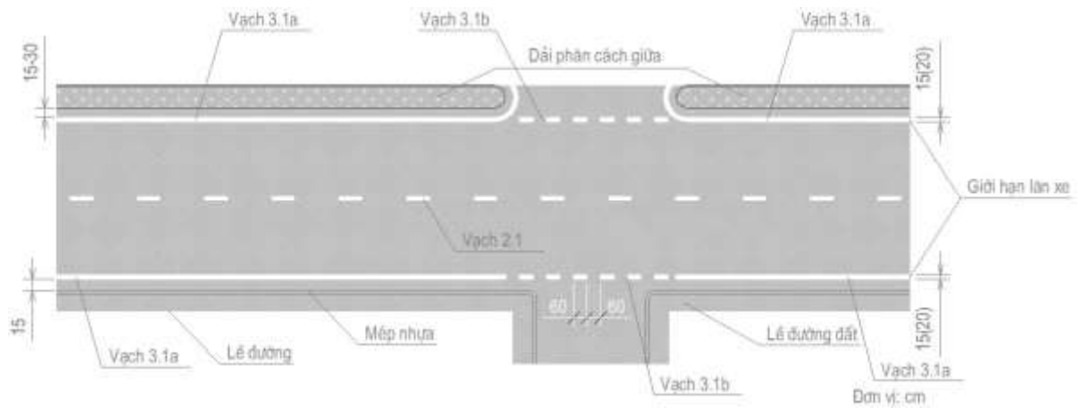
Hình G.13a - Minh họa sử dụng vach 3.1 để xác định mép ngoài phần xe chạy
