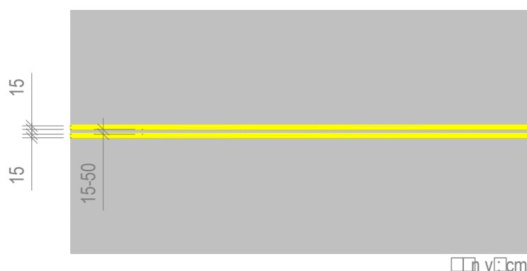
Hình G.3 - Vach 1.3
