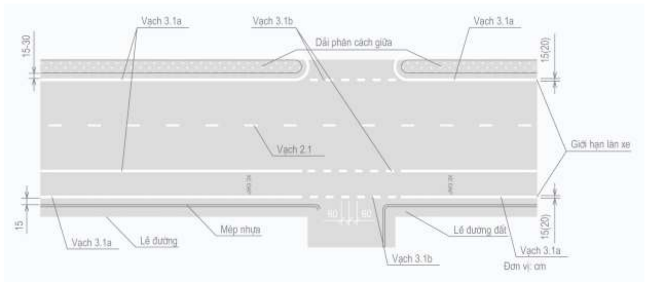
Hình G.13a - Minh họa sử dụng vach 3.1 để xác định mép ngoài phần xe chạy
