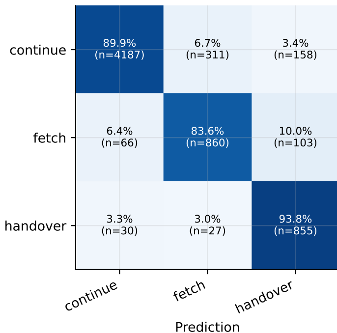
GRU
