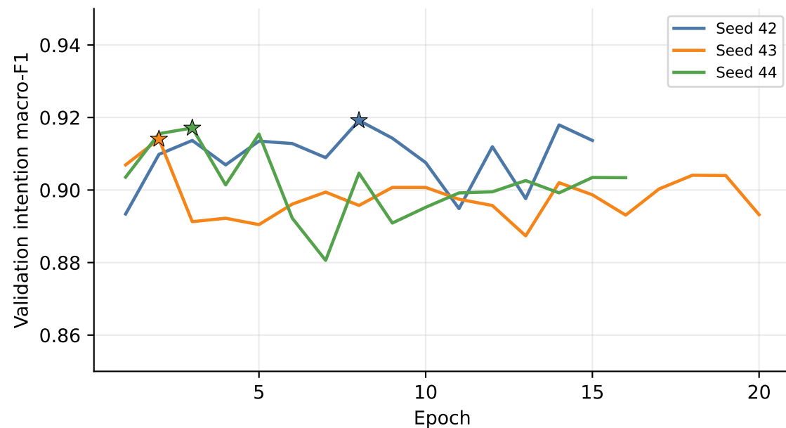
GRU
