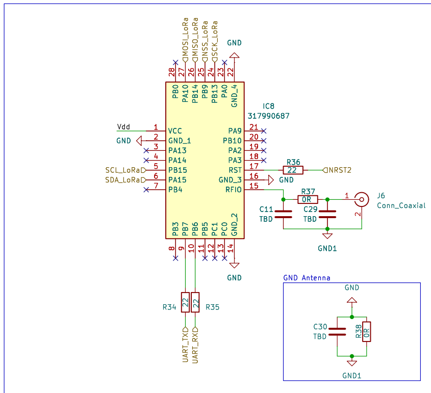
LoRa-E5 Module (Schaltung nach dem Referenzdesign Datenblatt S.15)
