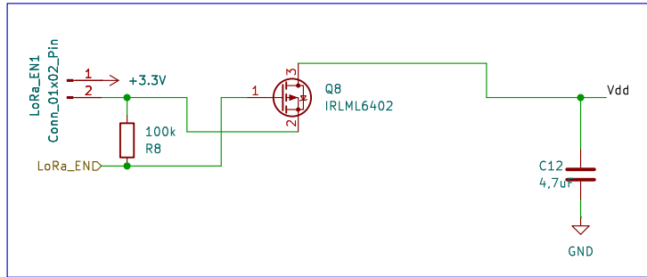
LoRa-E5 Module (Schaltung nach dem Referenzdesign Datenblatt Seite 15)
