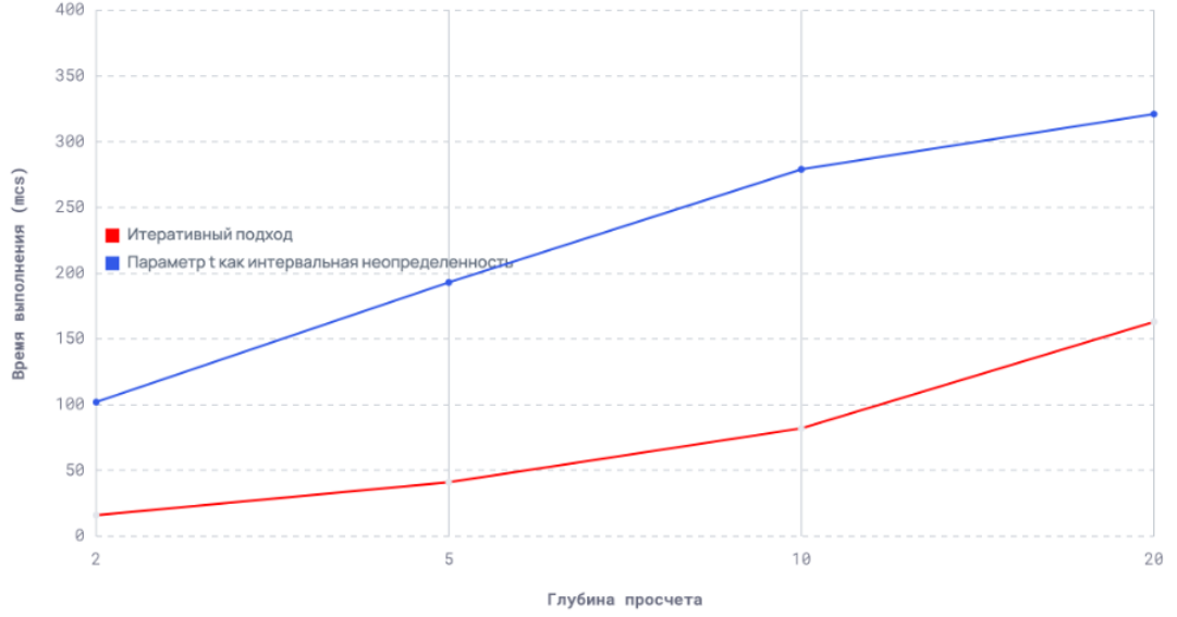
Рисунок 3 — Сравнение двух способов работы с двумерной динамической системой: t как дополнительная размерность и итеративный режим через MakeNextIteration
