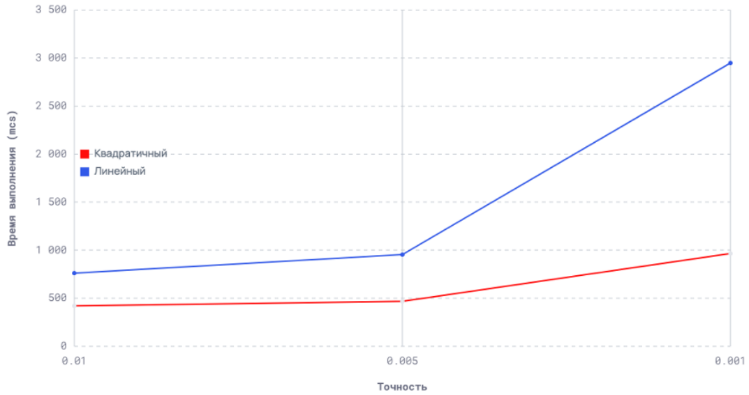
Рисунок 2 — Сравнение времени построения сетки для линейного и квадратичного базисов при различных значениях \varepsilon
