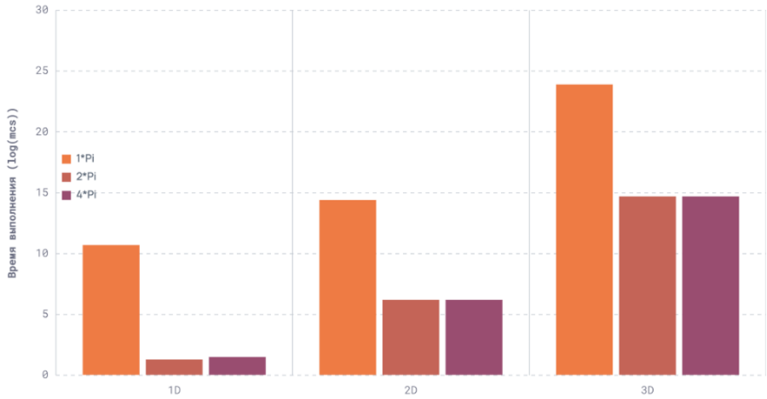
Рисунок 1 — Зависимость времени построения сетки от размерности задачи и размера области
