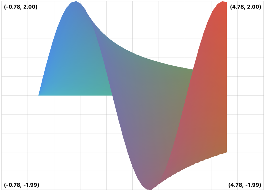
Рисунок 7 — Визуализация функции u = x , v = y(\sin(2.5x) + 0.35 \cos(6y) + 0.2 \sin(5x + 0.4) - 0.15 \cos(9y - 0.2)) во Flutter-клиенте
