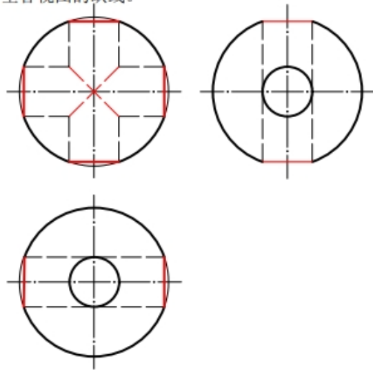
6-4 特殊相贯线、多立体表面相交
