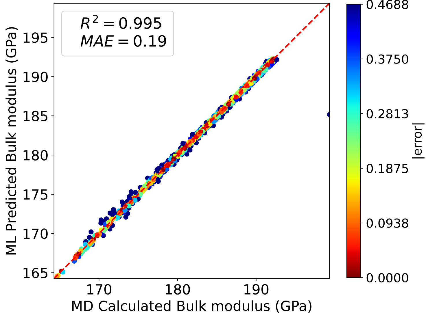
SGD (test)
