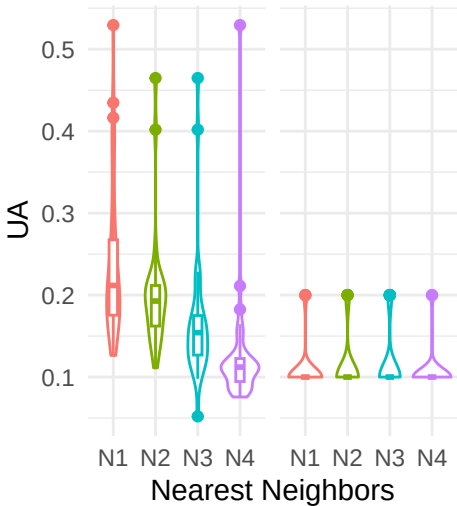
FunCN
