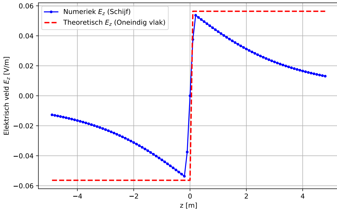
Elektrisch veld op de z-as ( r = 0 )
