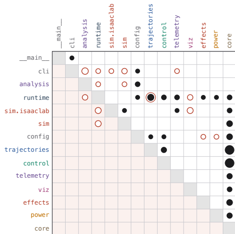
b 设计结构矩阵 (DSM)
