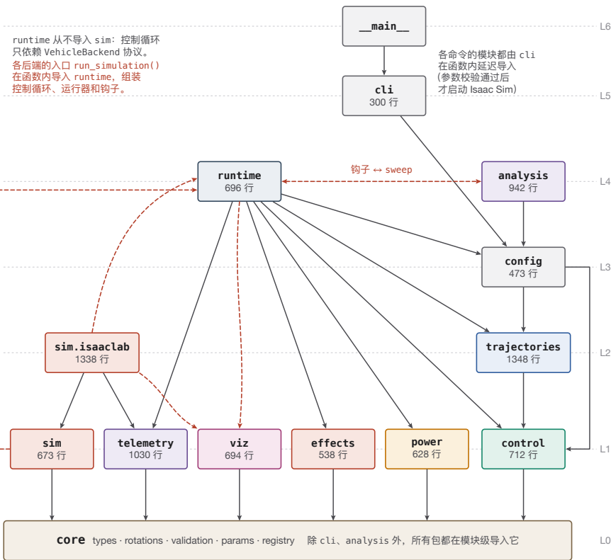
a 模块级导入构成一个以 core/ 为底的有向无环图
